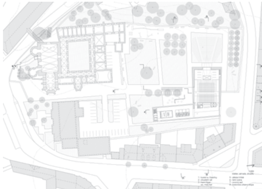
Divadelní sál, klášterní zahrada, půdorys
