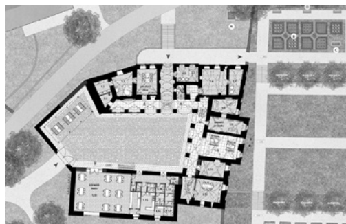
Půdorys přízemí, návrh revitalizace
