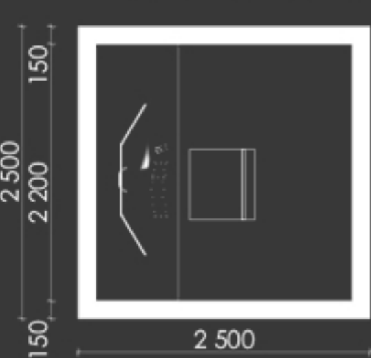
PŮDORYS M 1:25
