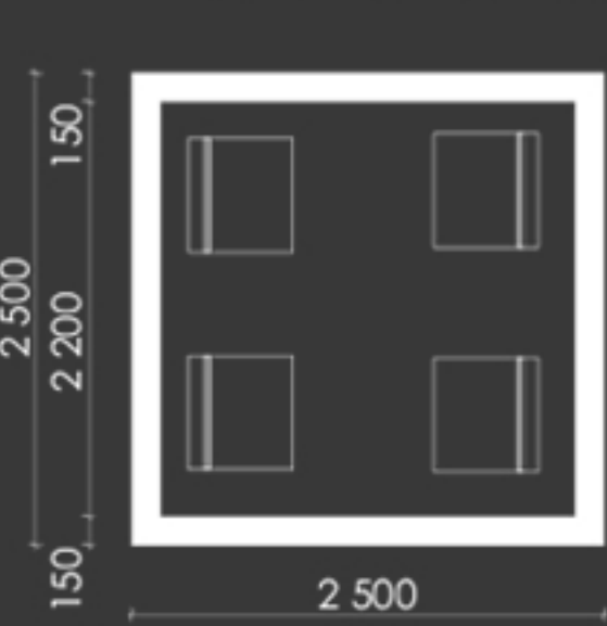
PŮDORYS M 1:25
