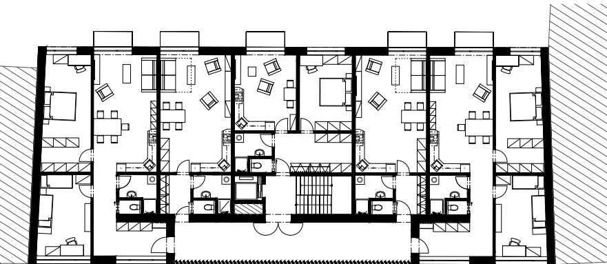
Půdorys typického podlaží
