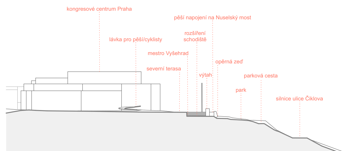
příčný řez severní terasou
