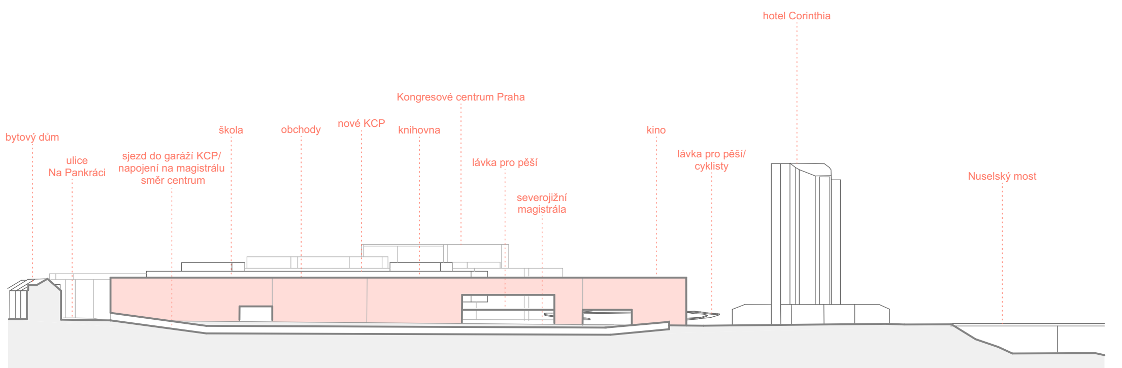
podélný řez jižní terasou
