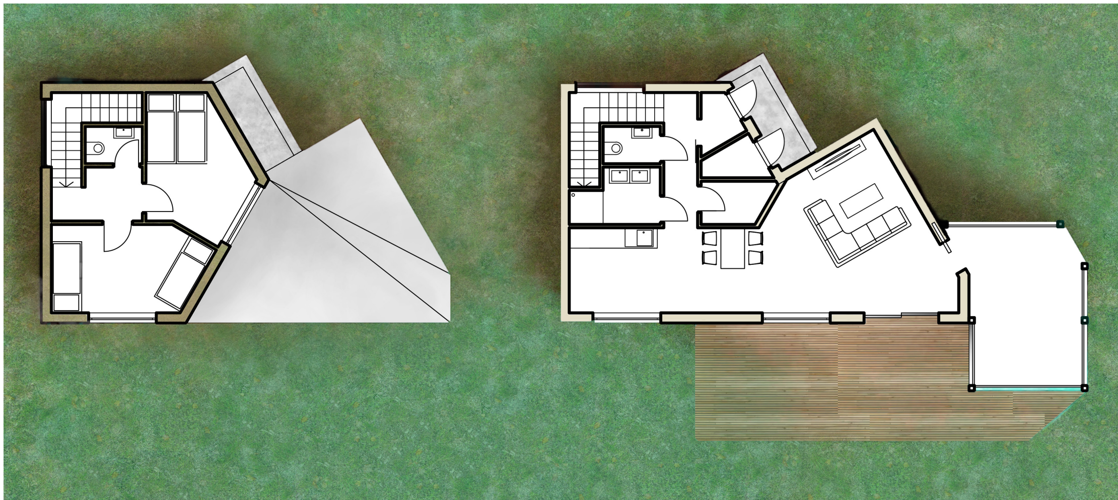
PÔDORYS A 1NP, 2NP
