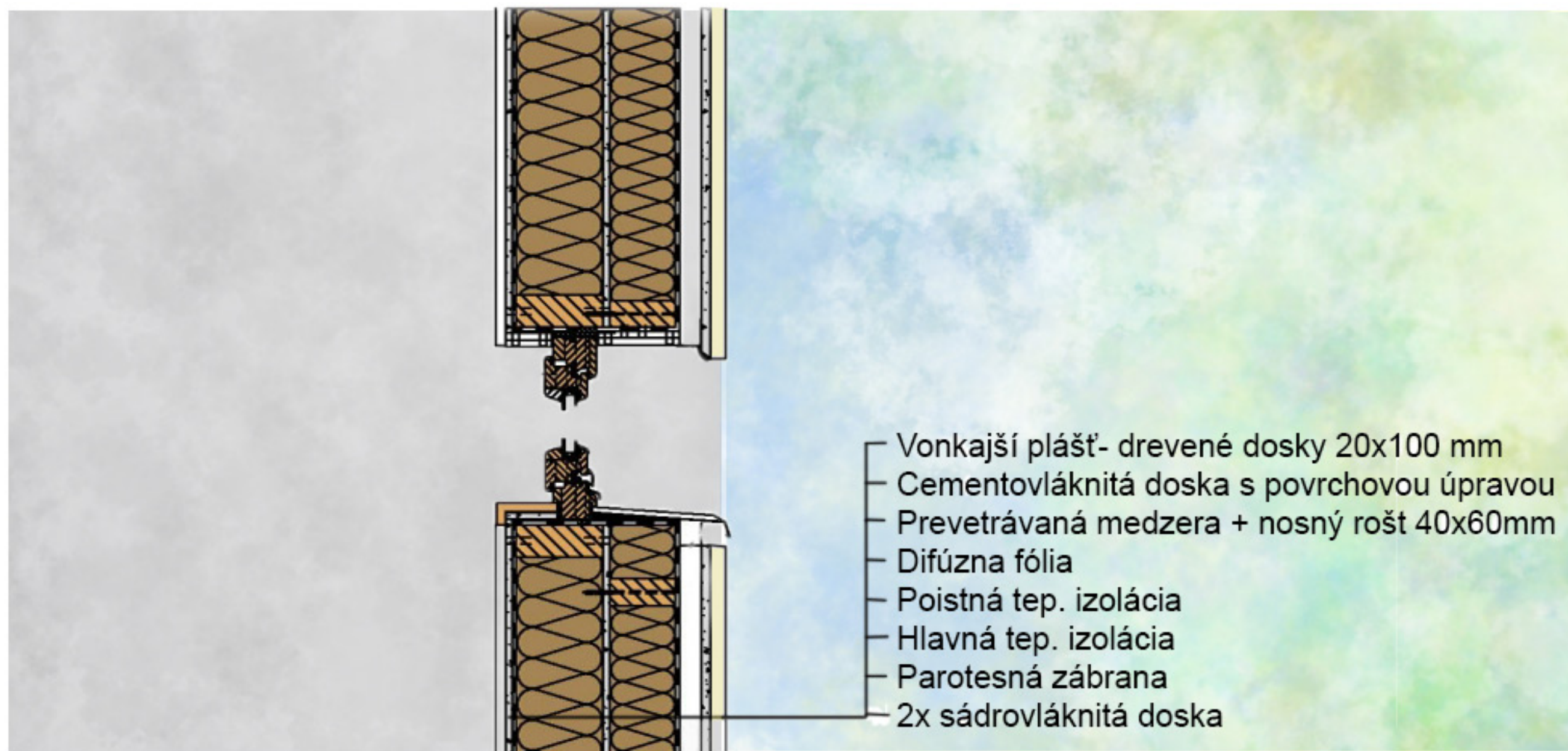
DETAIL OKNA
