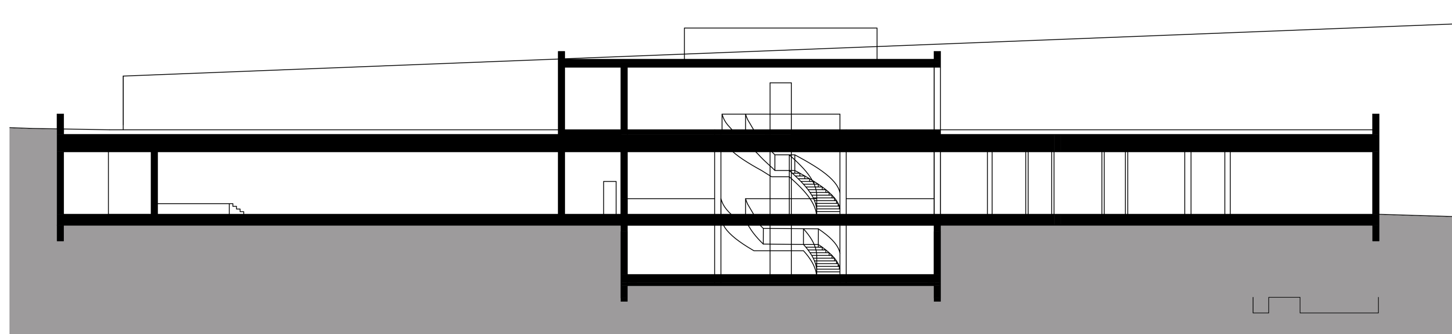
ŘEZ PODÉLNÝ
