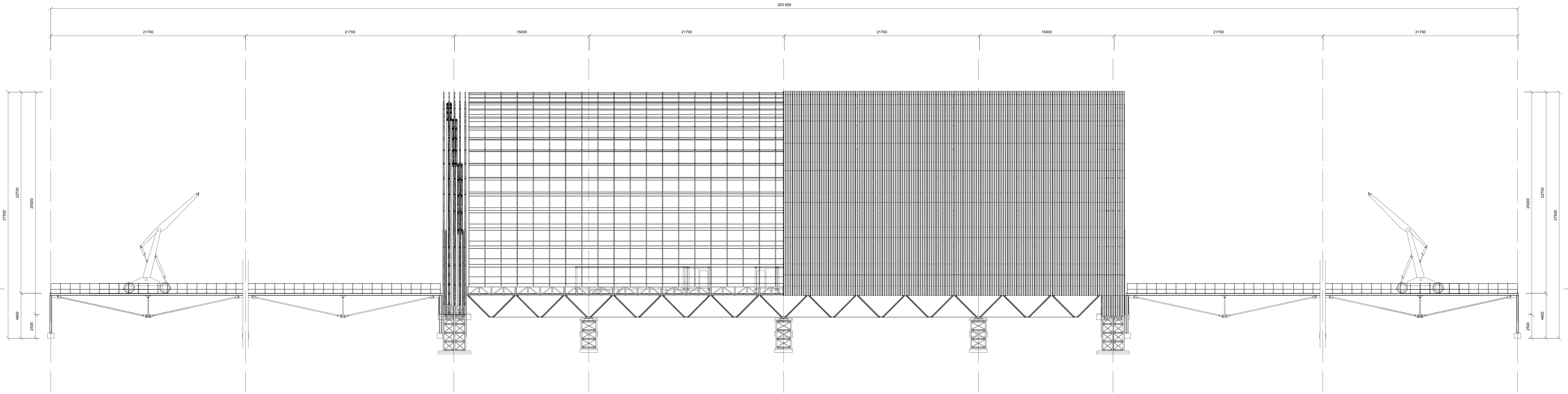
Pohled Zobrazení částečně rozložené konstrukce
