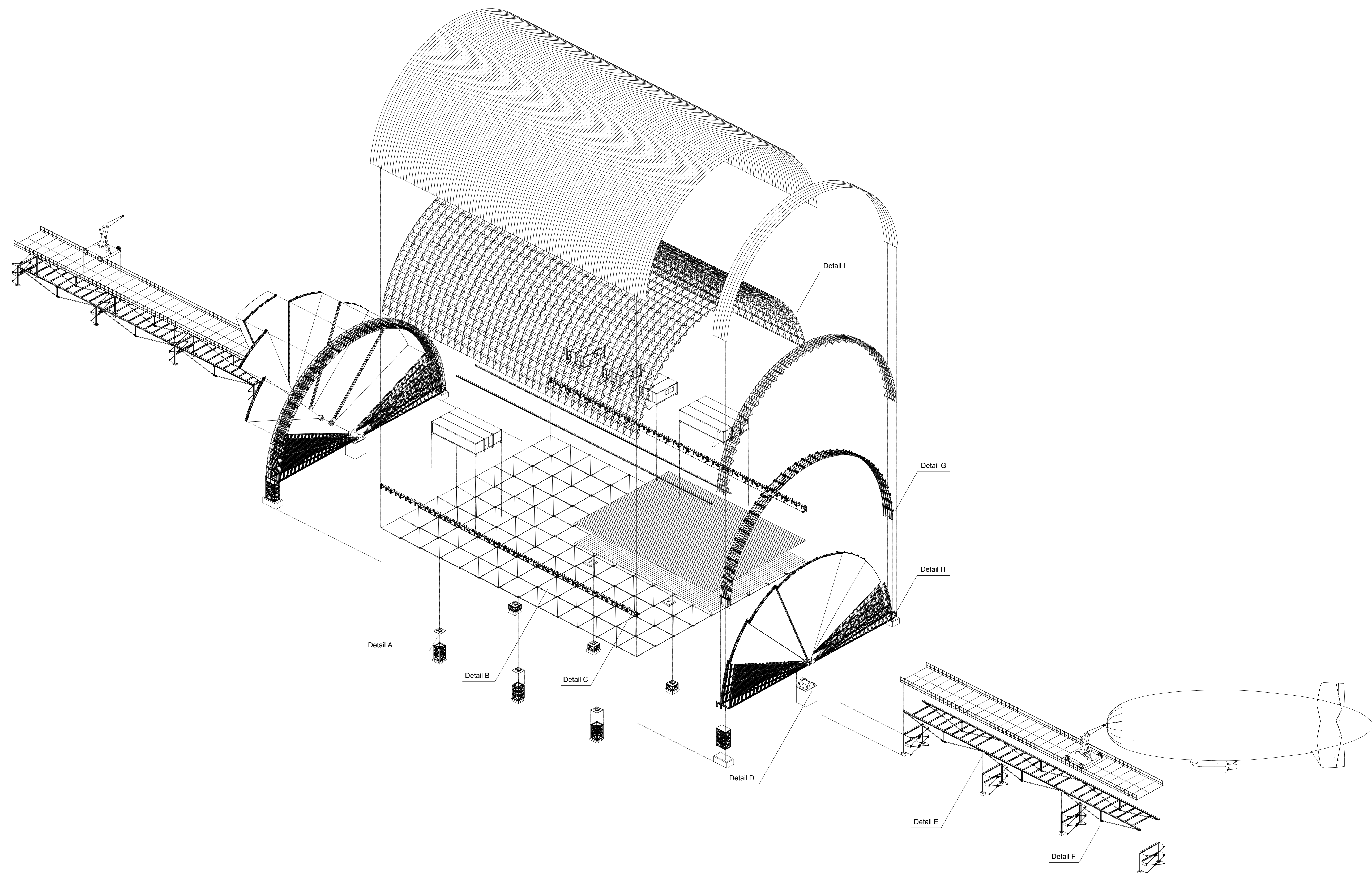
Axonometrie Rozložená konstrukce hangáru
