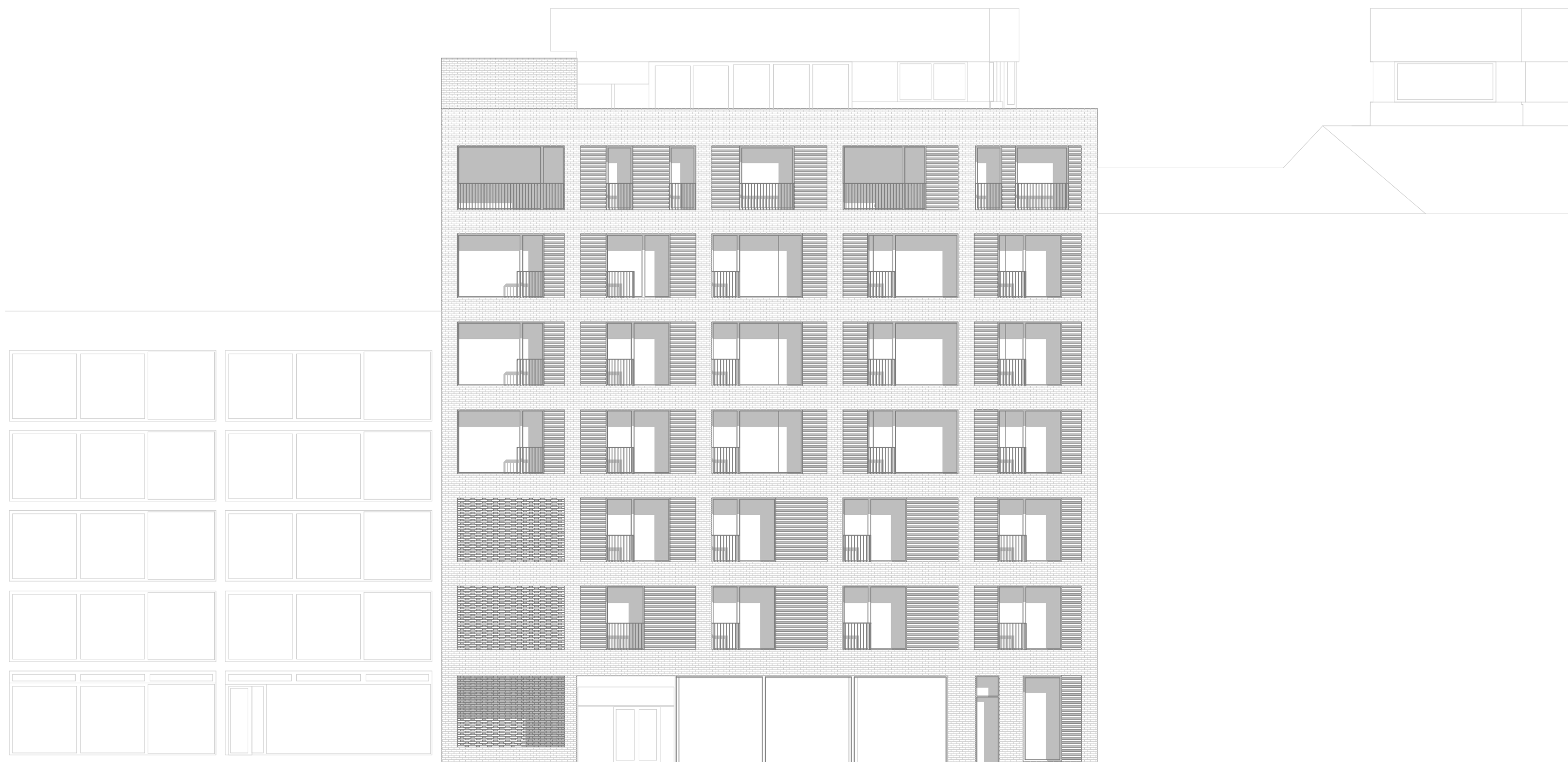
ZÁPADNÍ POHLED
