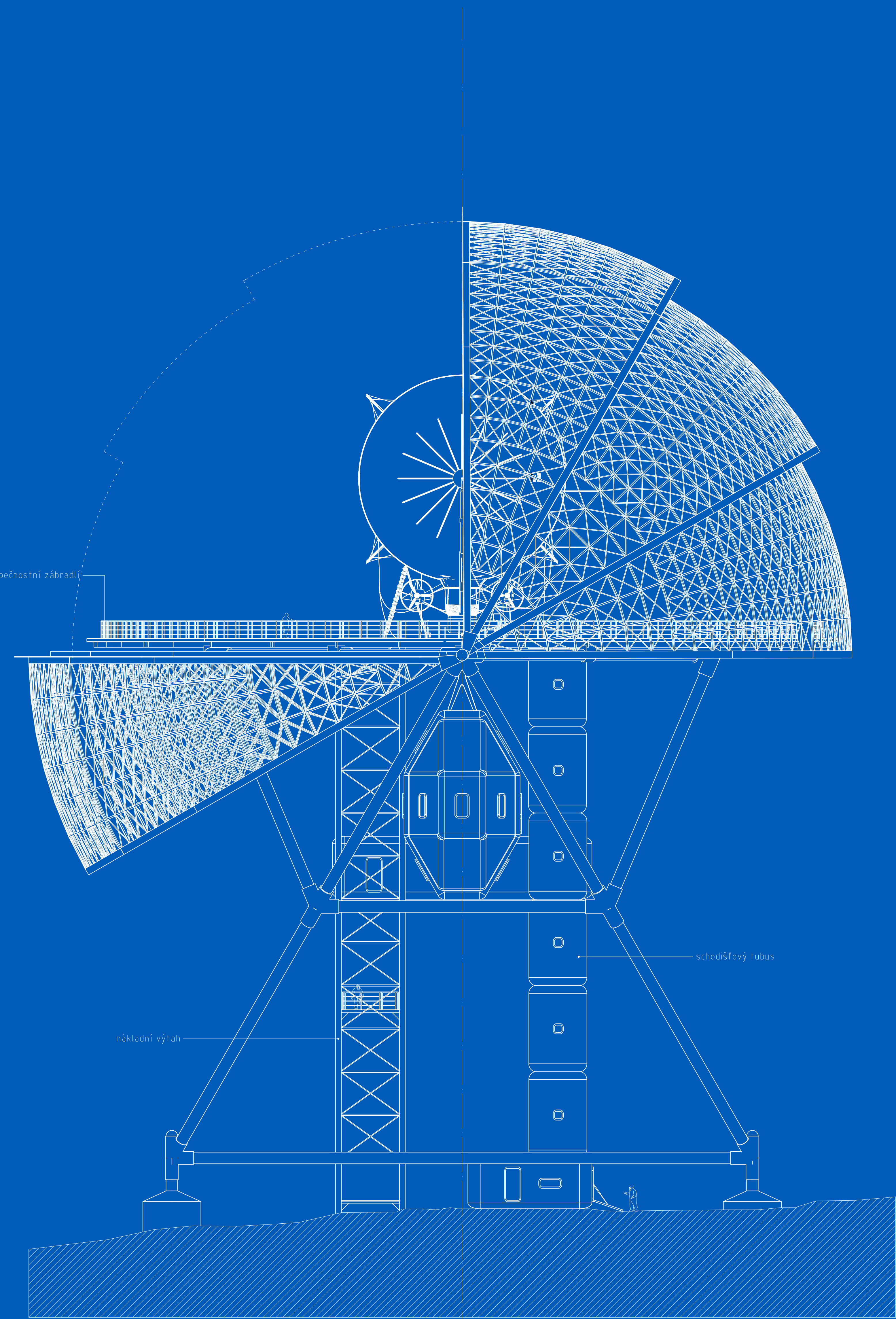
příčný pohled _ otevřeno - zavřeno _ m 1:150
