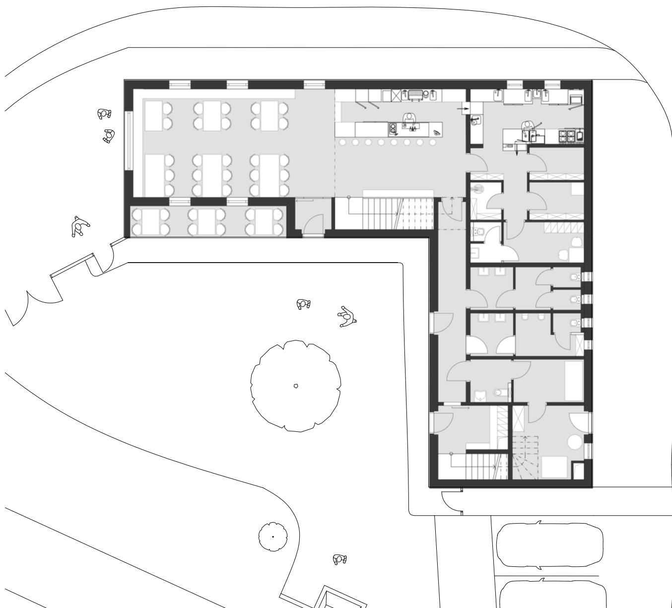
PŮDORYS PŘÍZEMÍ
