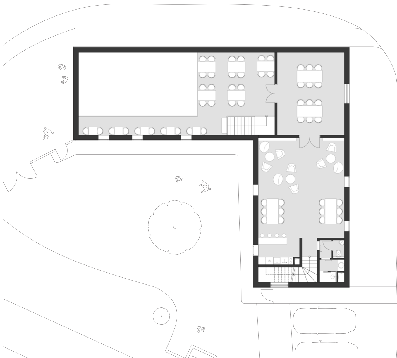
PŪDORYS PATRA
