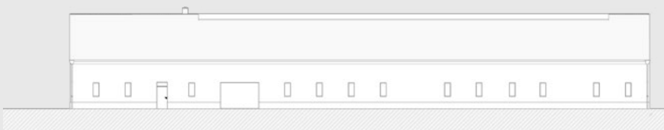
VÝCHODNÍ FASÁDA
