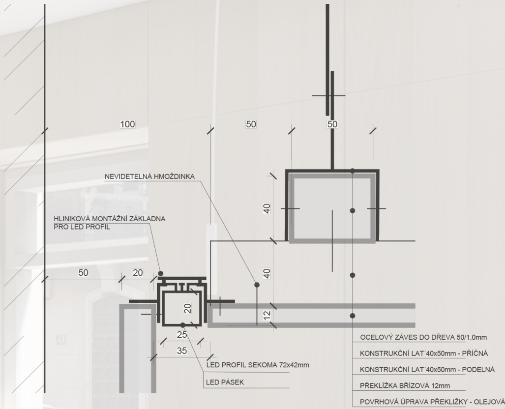
DETAIL 1: NAPOJENÍ PODHLEDU NA STĚNU
