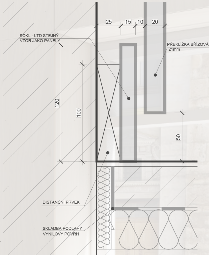
DETAIL 3: UKONČENÍ U PODLAHY
