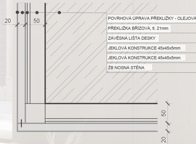
DETAIL 1: NAPOJENÍ NA OKNO
