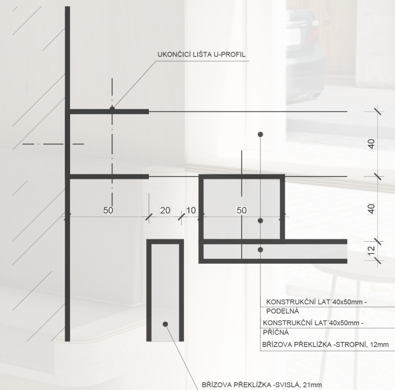
DETAIL 1 - ŘEZ
