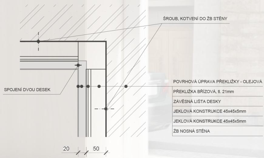
DETAIL 2: NAPOJENÍ NA ROHU
