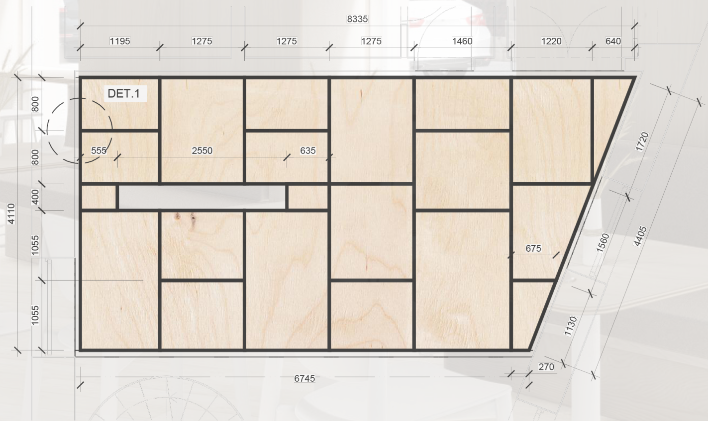
PŮDORYS PODHLEDU - PANELY
