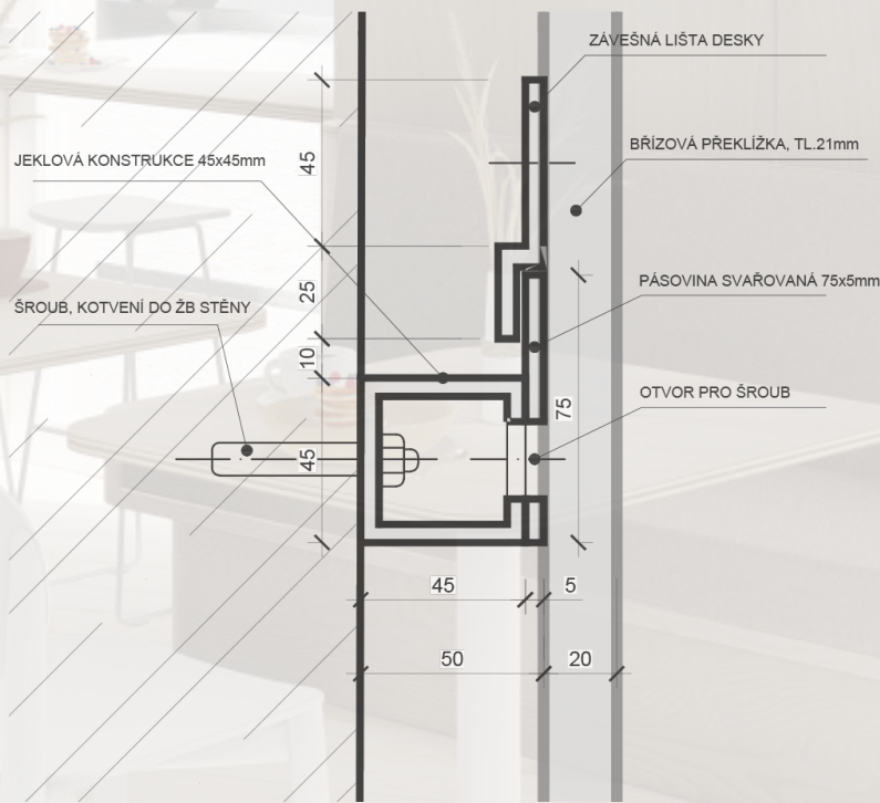
DETAIL 2: ZAVEŠENÍ PANELU NA STĚNU
