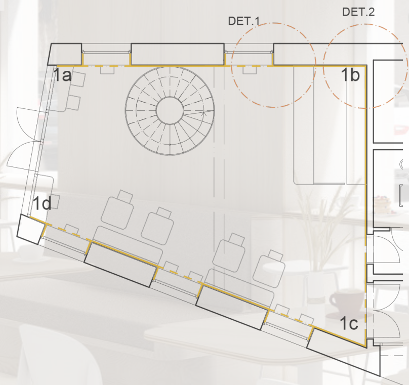
PŮDORYS PŘÍZEMÍ
