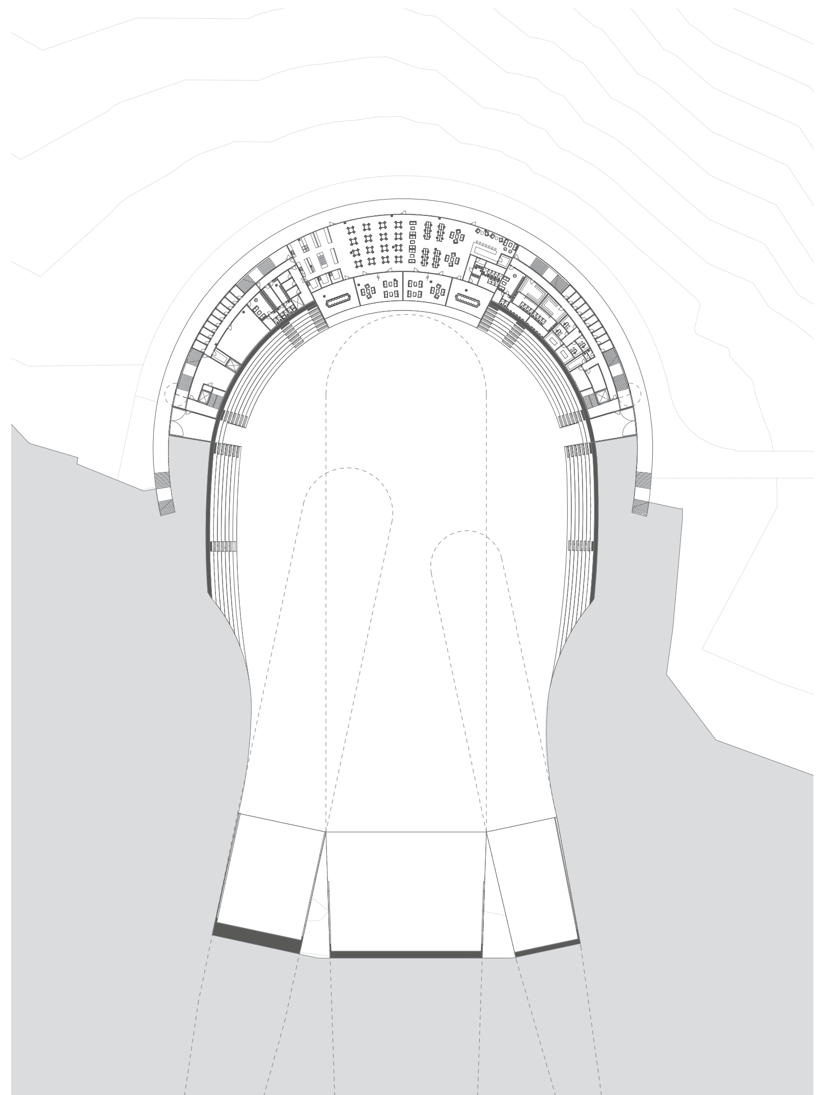
Pådorys 1.NP
