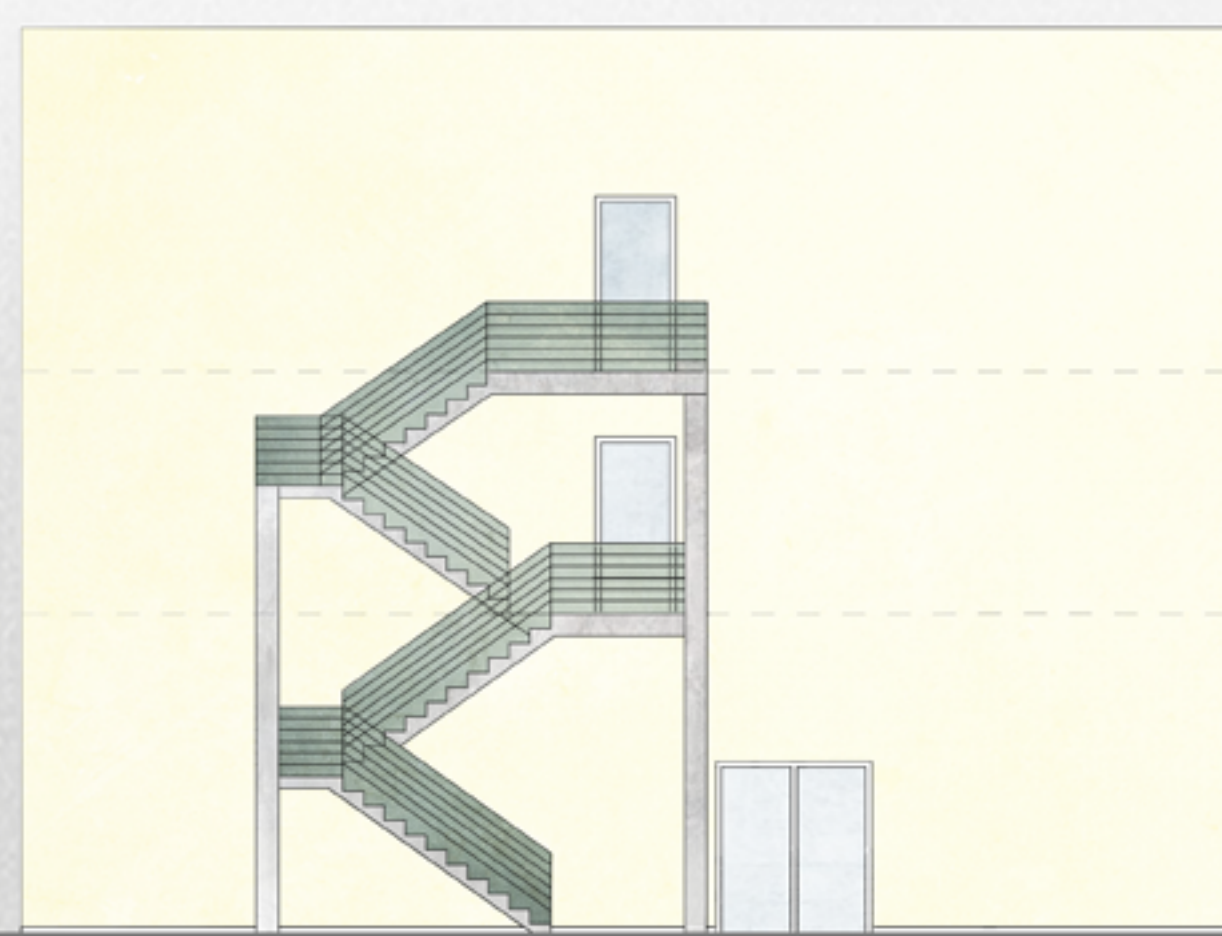
POHLAD VÝCHOD 1:100
