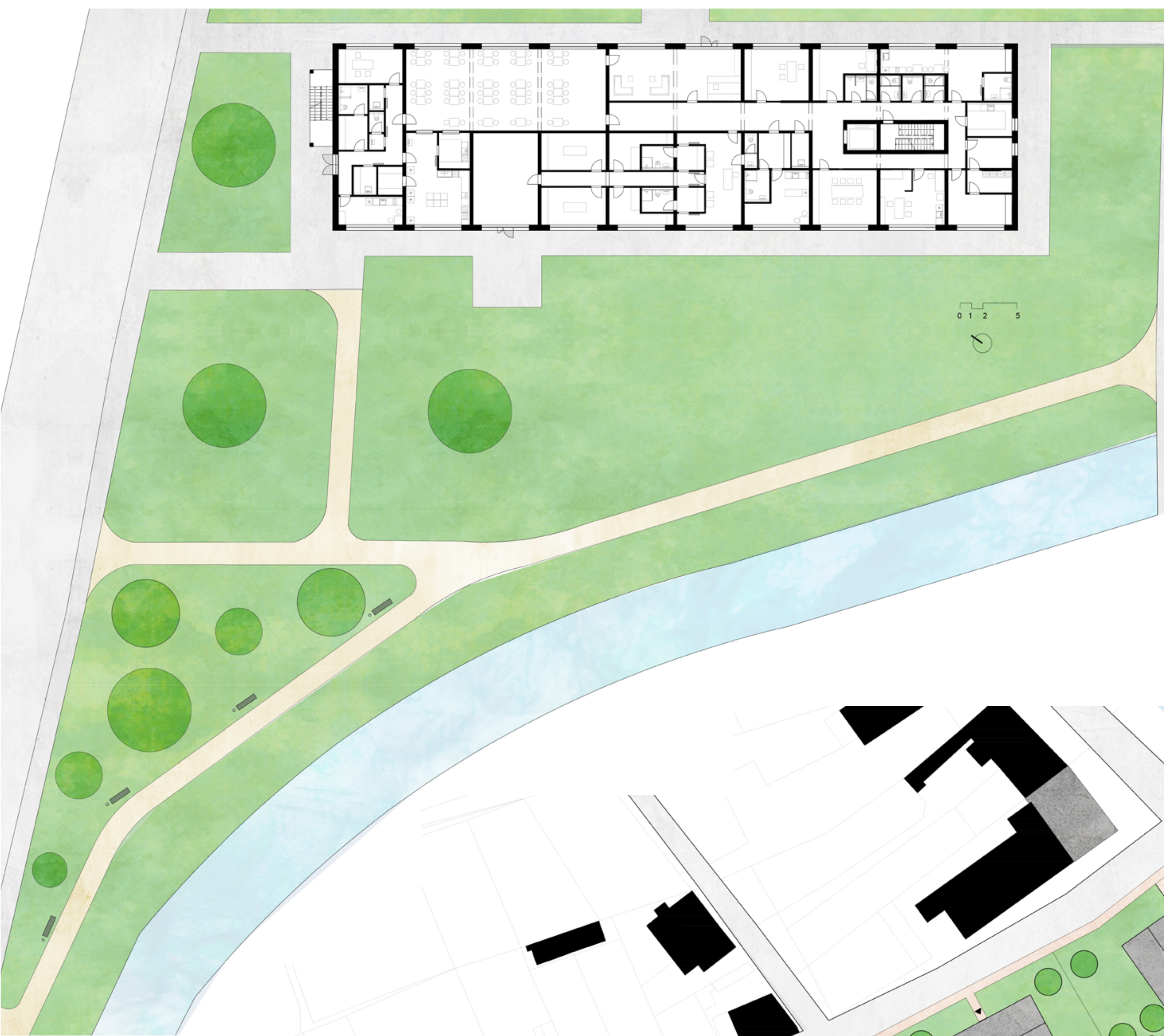
PŮDORYS 1NP 1:200
