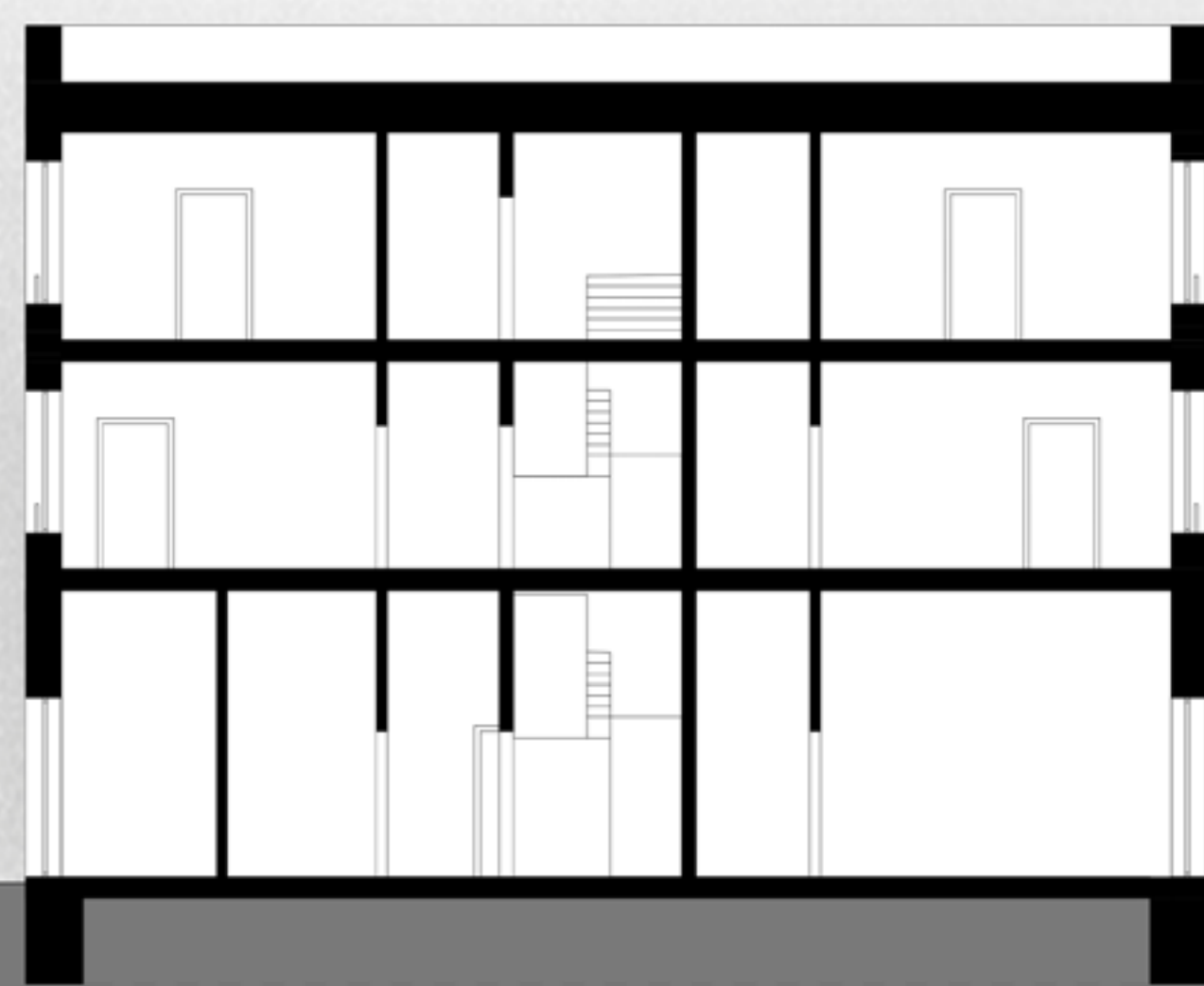
REZ 1:100
