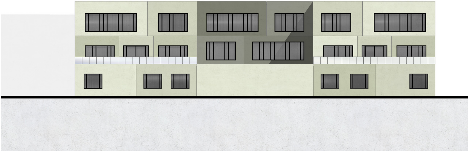
Západný pohľad
