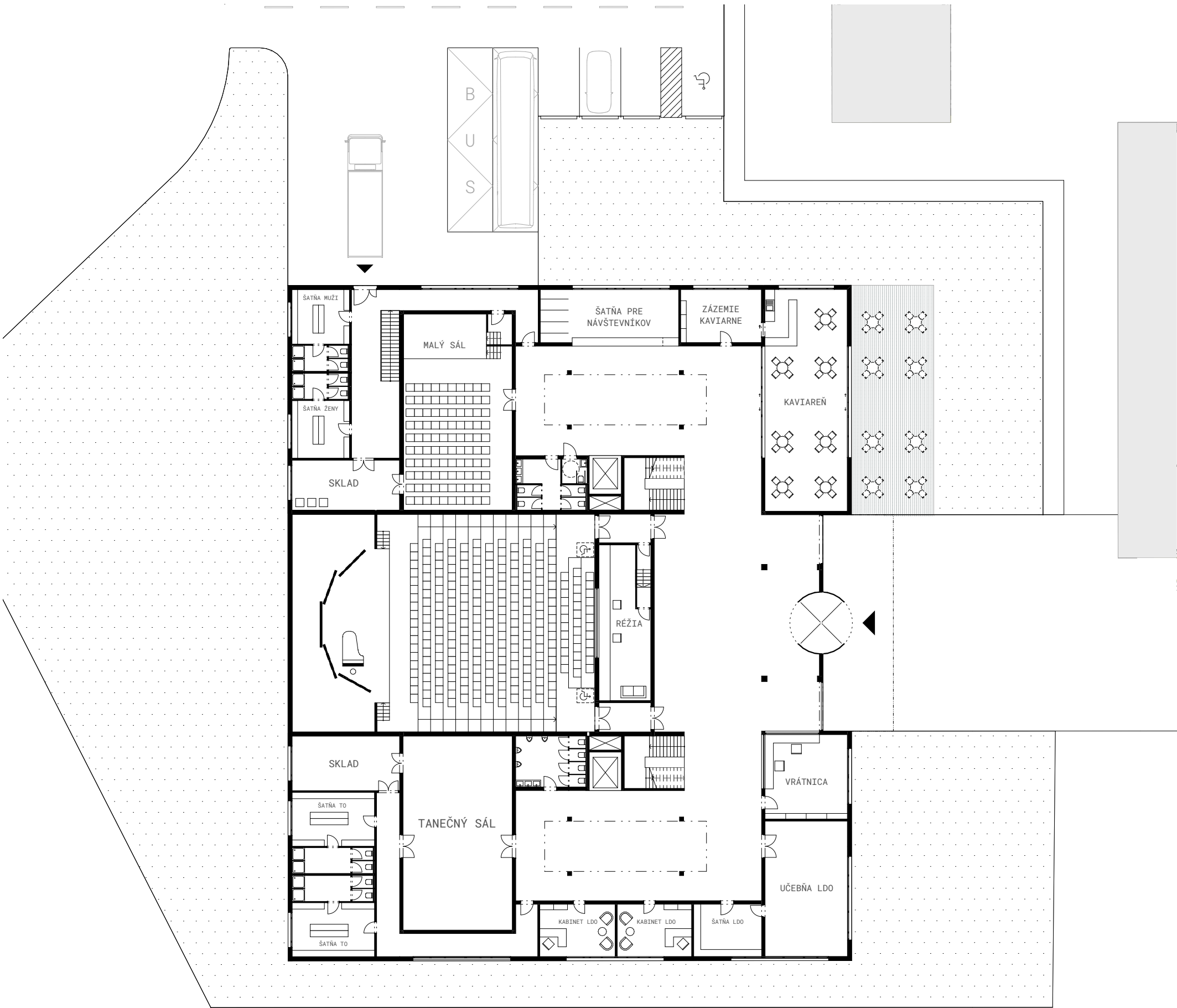
pôdorys 1.NP
