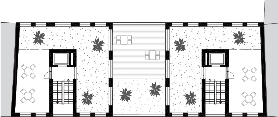
Půdorys 5np
