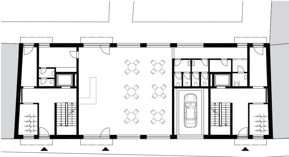
Půdorys parteru v Jindřišské
