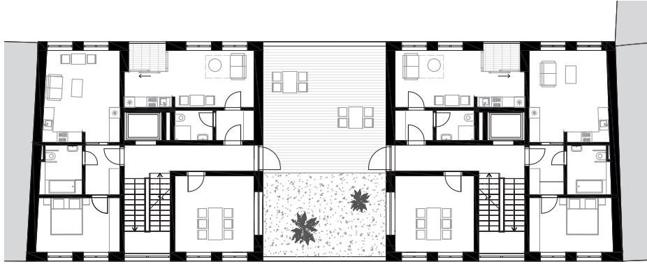
Půdorys 2np - 4np
