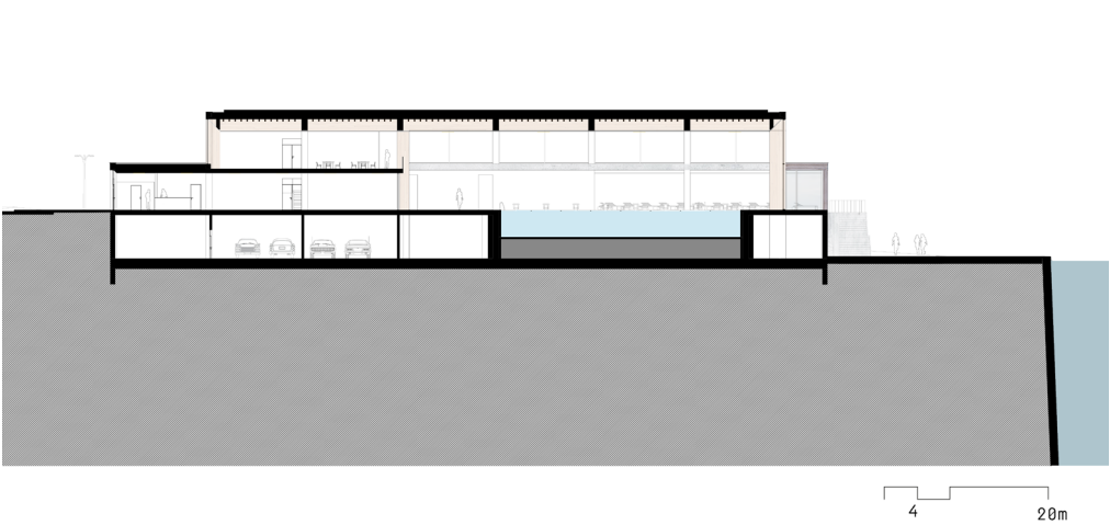
Řez 2
