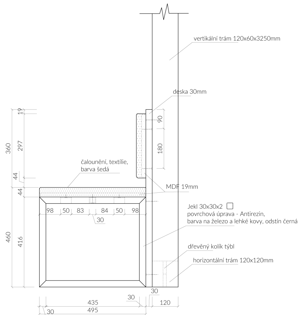
POHLED BOČNÍ 1:10
