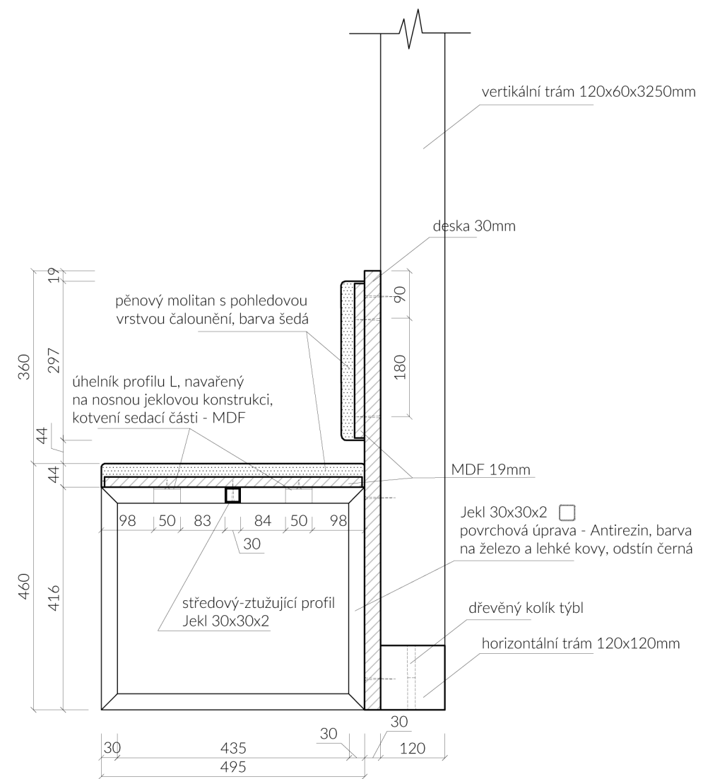
ŘEZ 1:10
