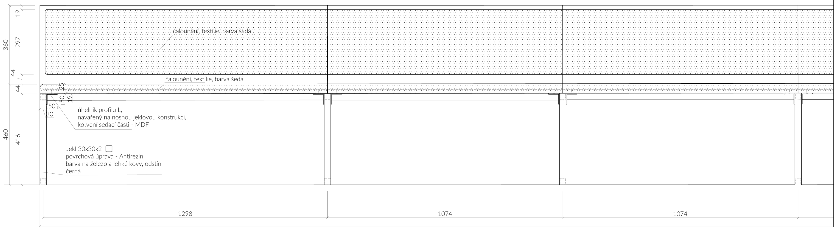
POHLED ČELNÍ 1:10
