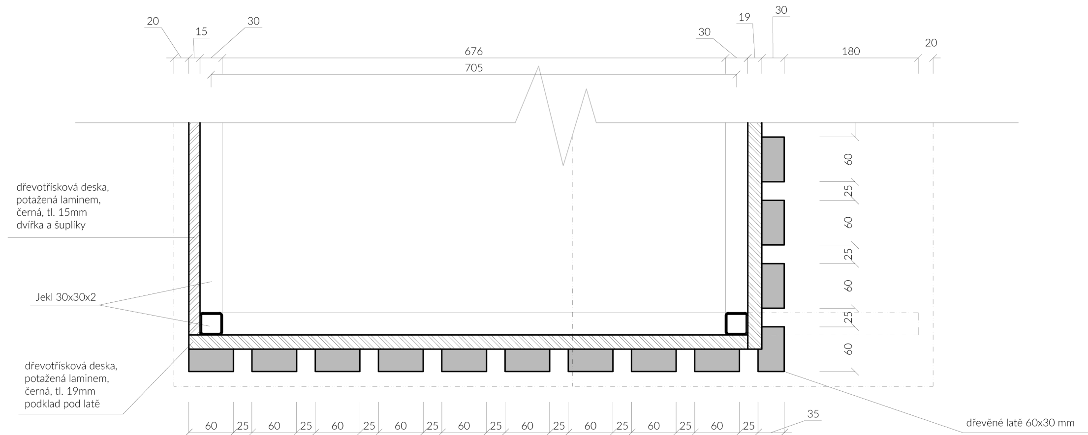
OBLOŽENÍ BARU LATĚMI 1:5
