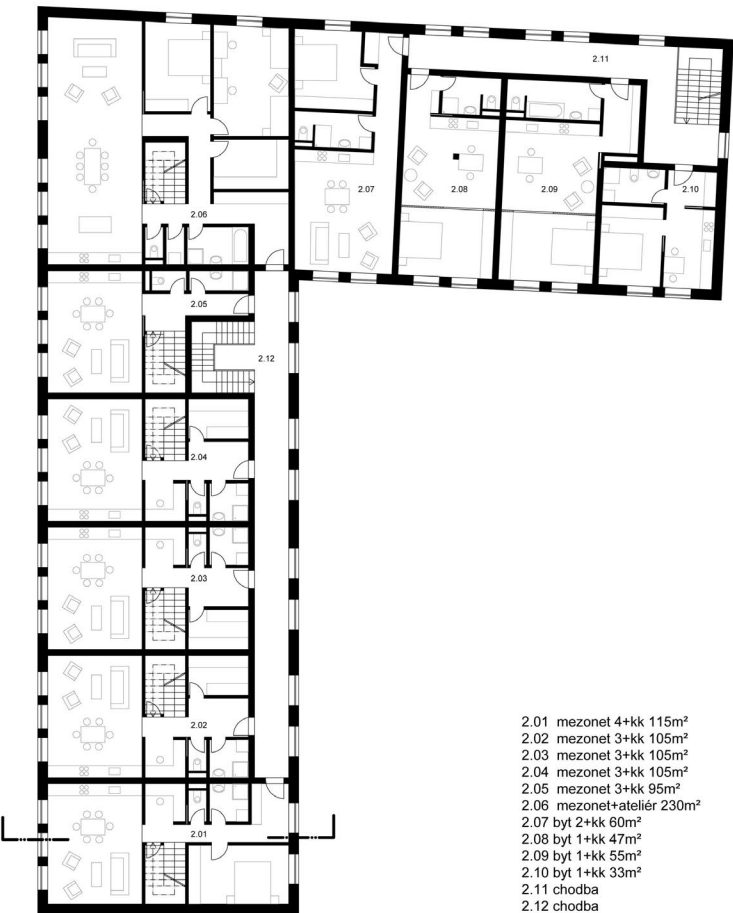
PŮDORYS 2NP 1:200
