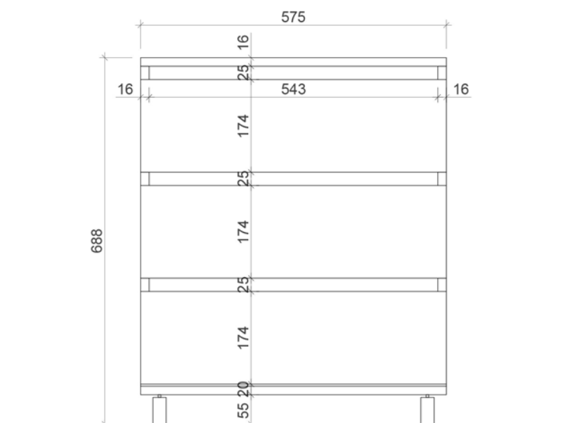
POHLED
