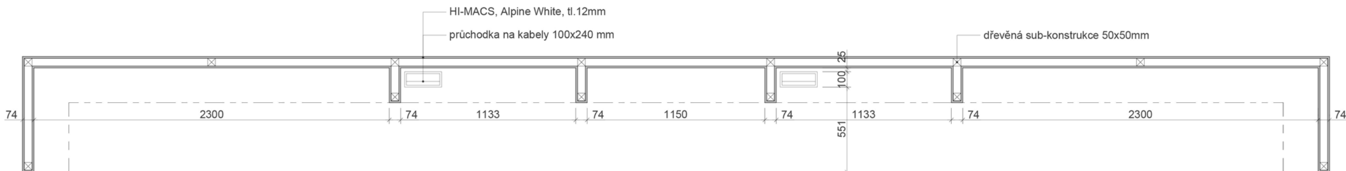
ŘEZ B-B
