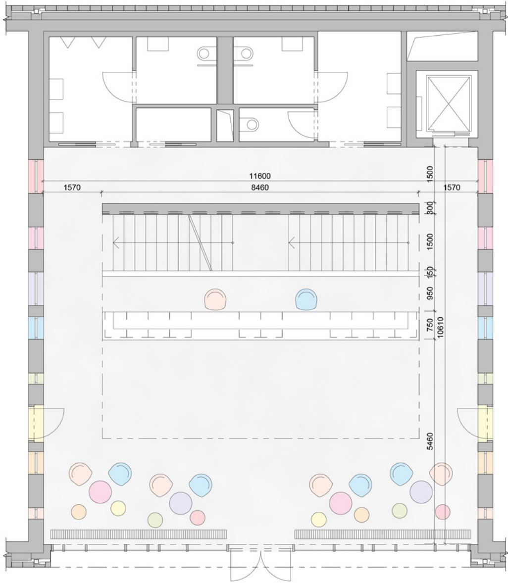
1NP
