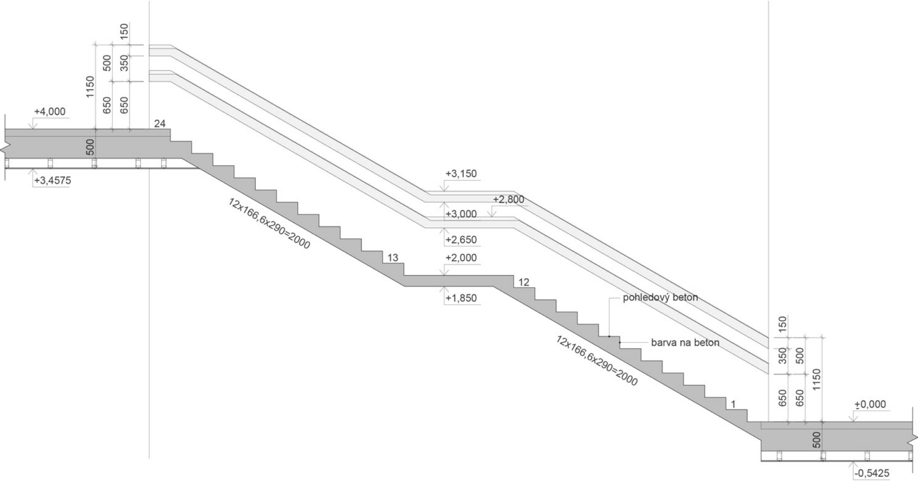
ŘEZ A-A'
