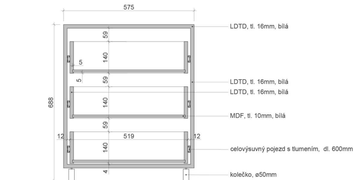
ŘEZ B-B'
