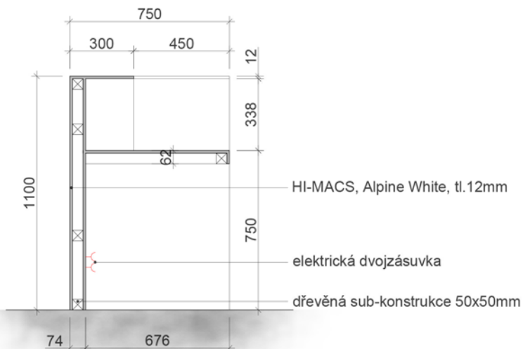
ŘEZ A-A
