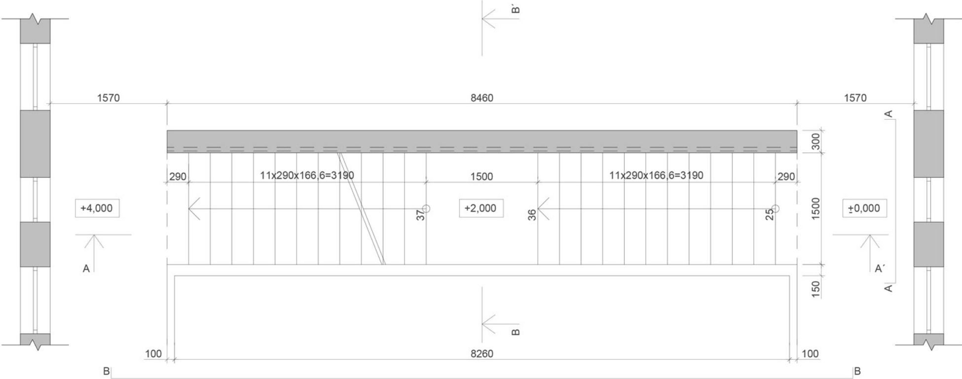
PŮDORYS
