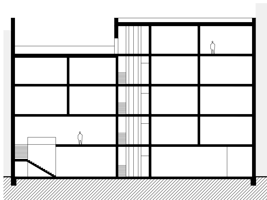
Řez podélný
