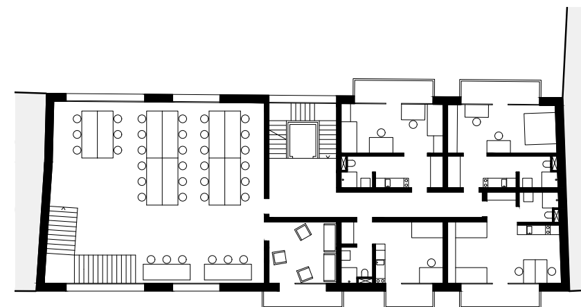
Půdorys 2np
