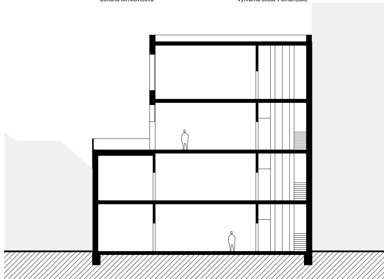
Řez A-A'
