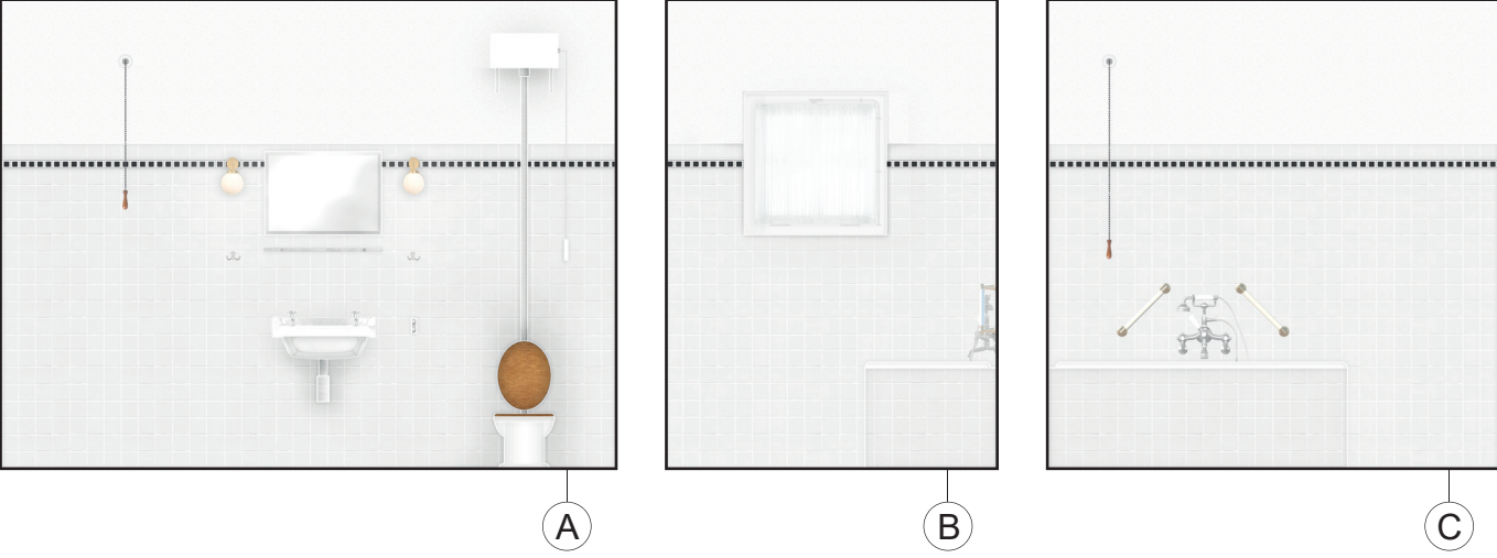
POHLEDY NA STĚNY M 1:50
