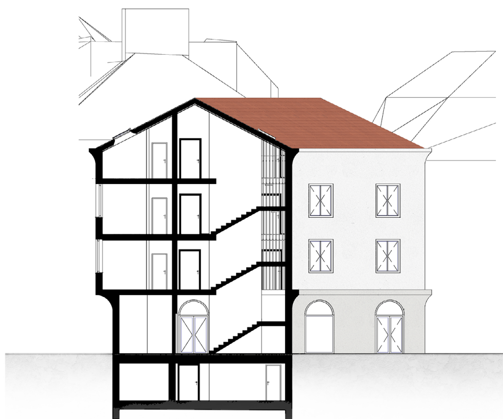
řez schodištěm
