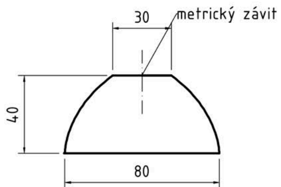
Půdorys
