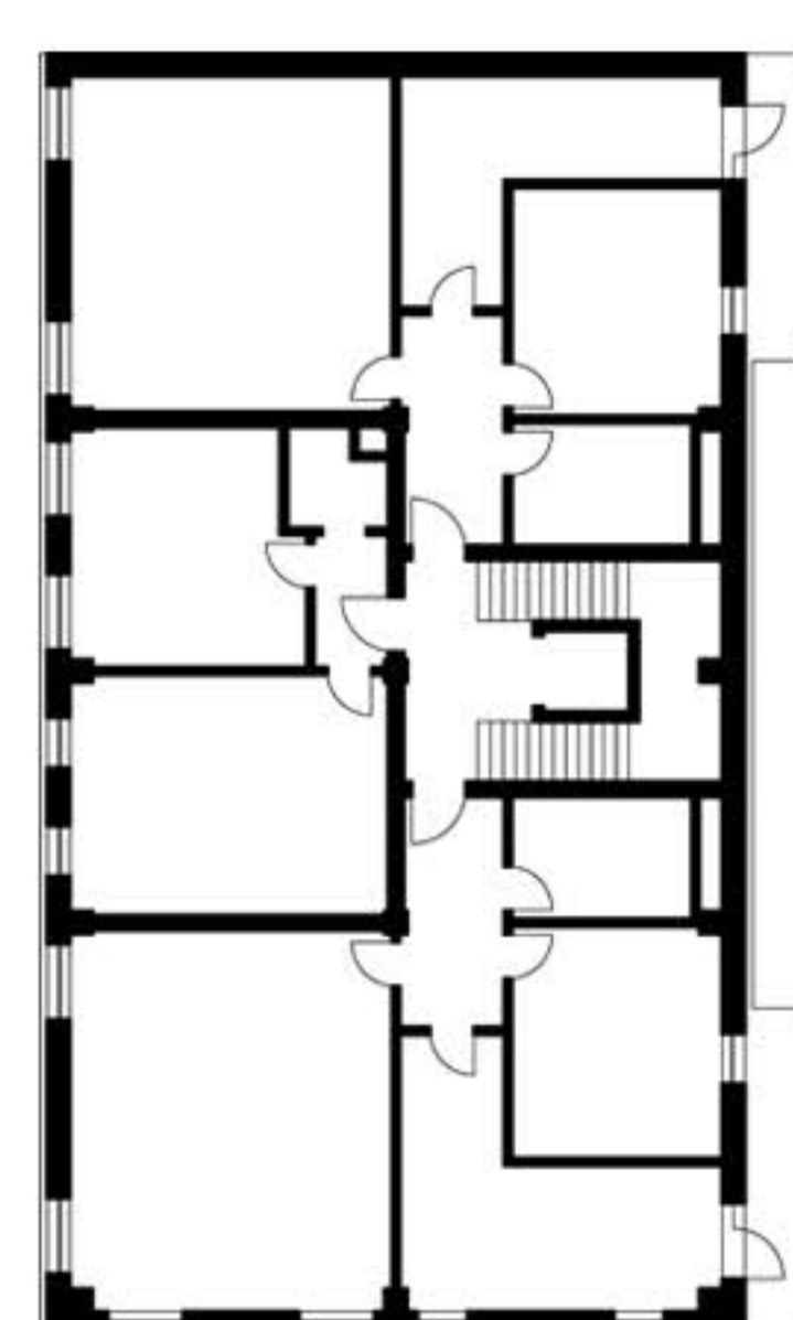
PŮDORYS TYPICKÉHO PODLAŽÍ
