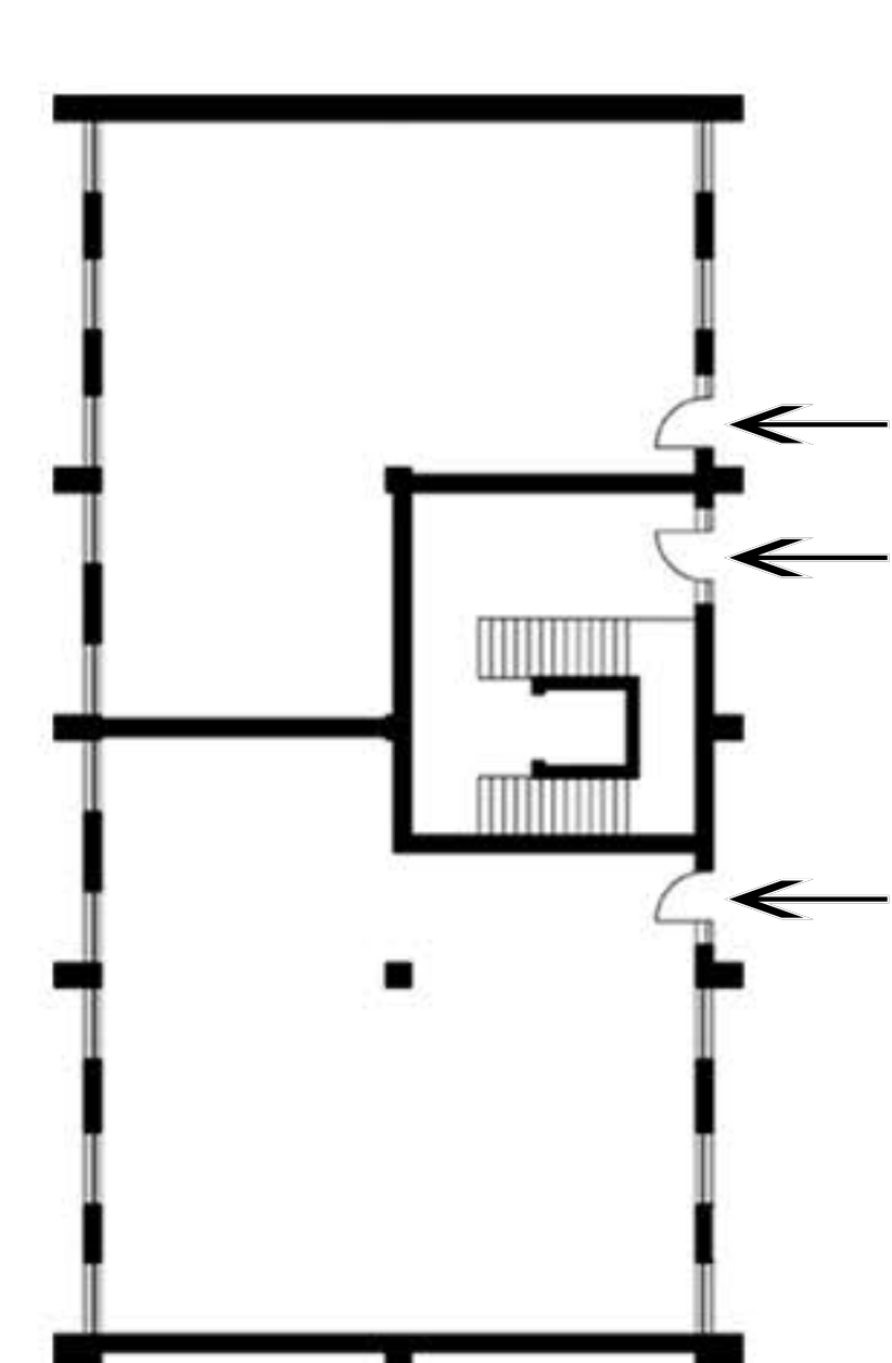
PŮDORYS PARTERU
