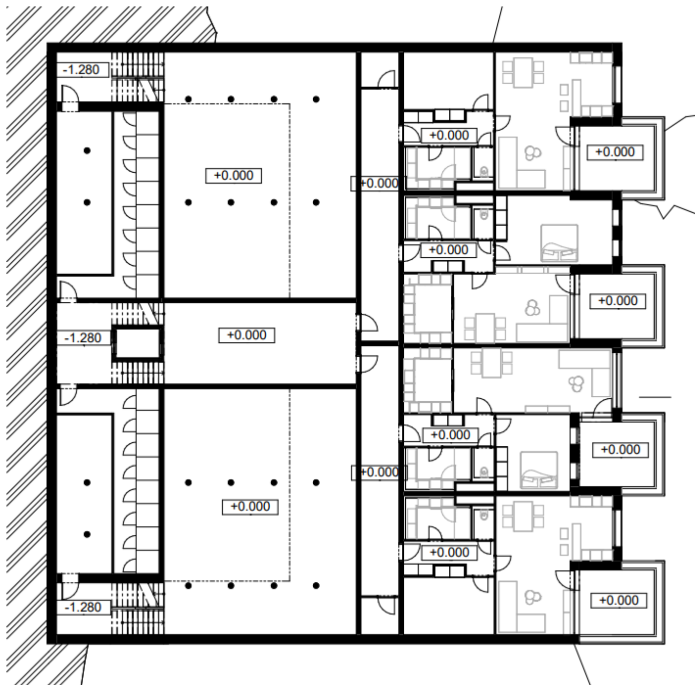
1.NP 1:200
