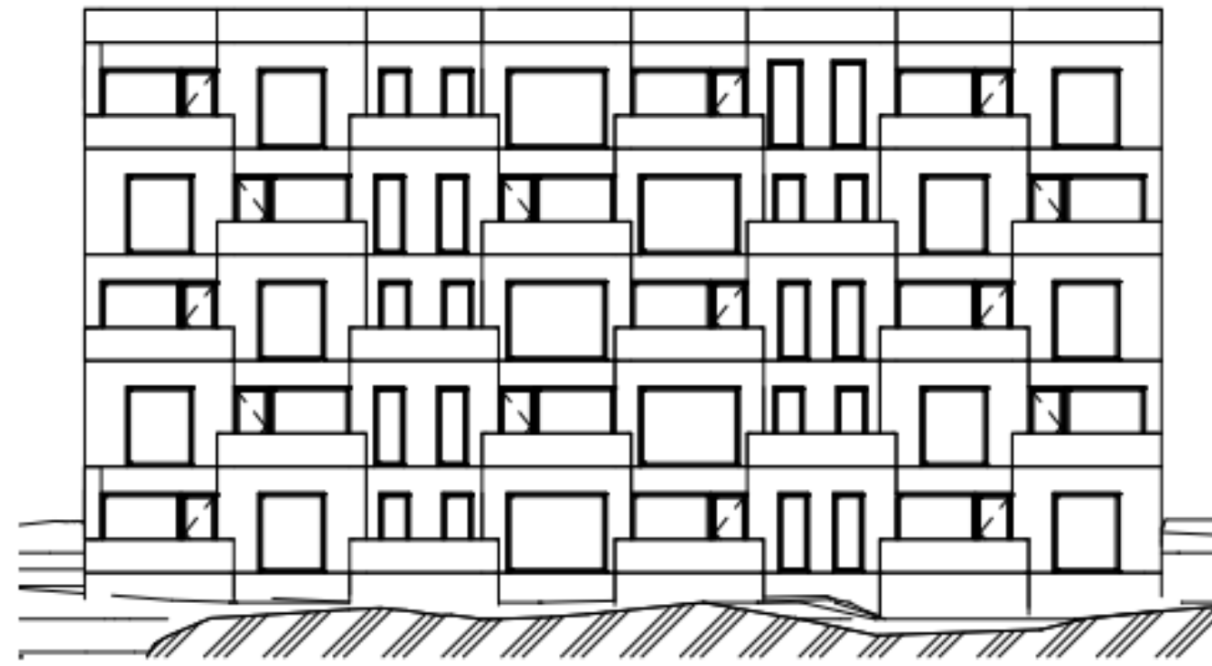
POHLED JIŽNÍ 1:200
