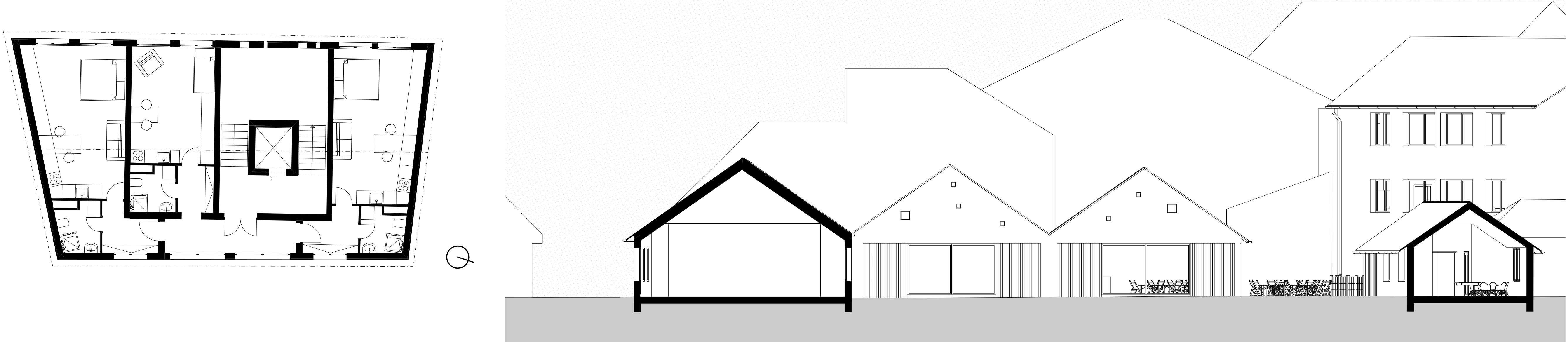
POHLED BD 1:100
