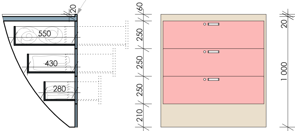
ŘEZ A
