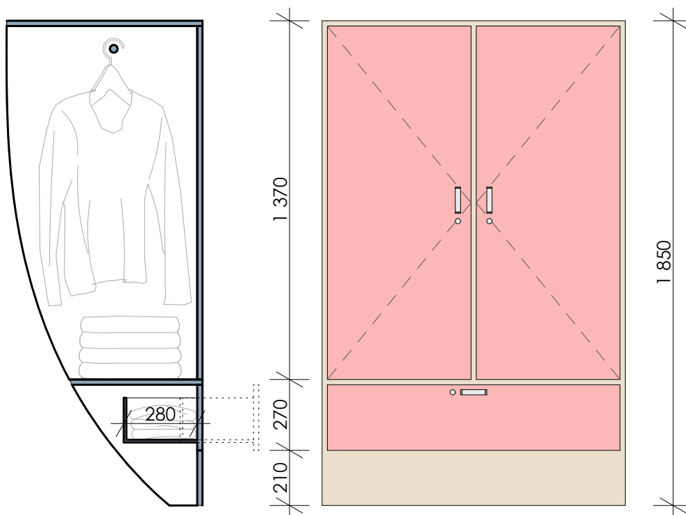
ŘEZ A
