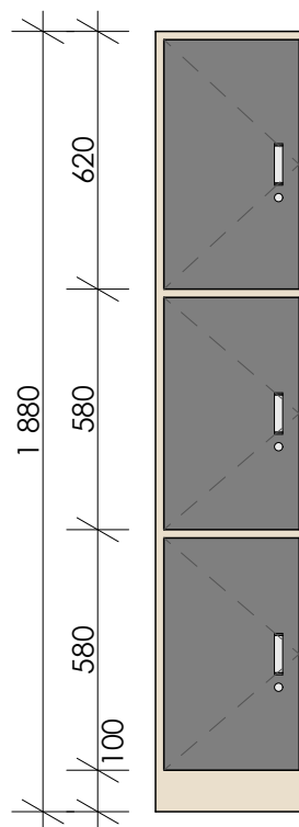
ČELNÍ POHLED
