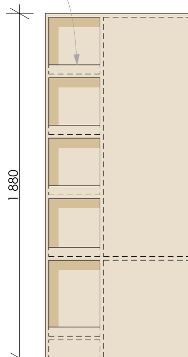
POHLED B
