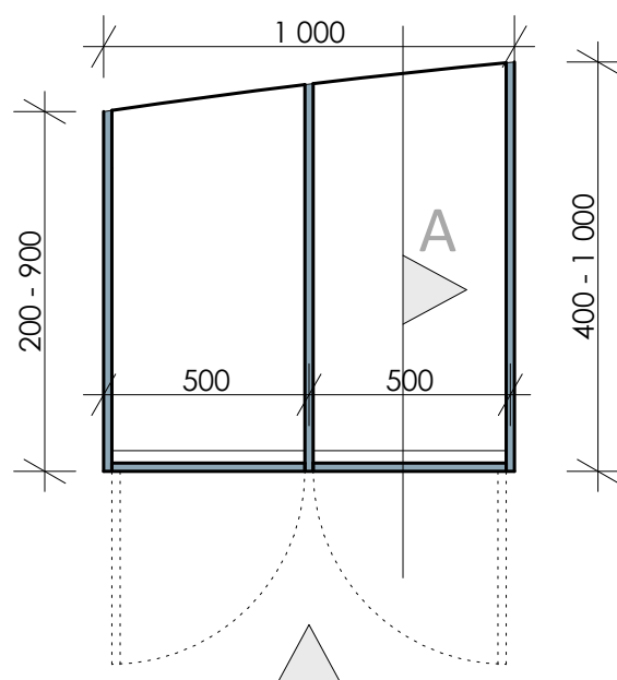
PŮDORYS
