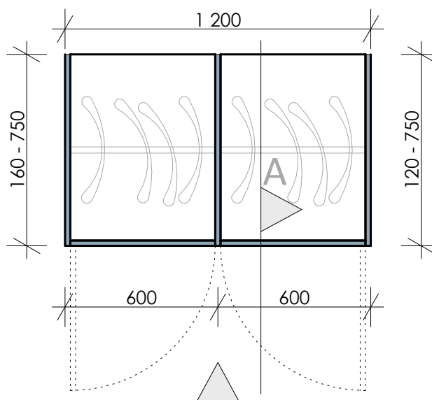
PŮDORYS
