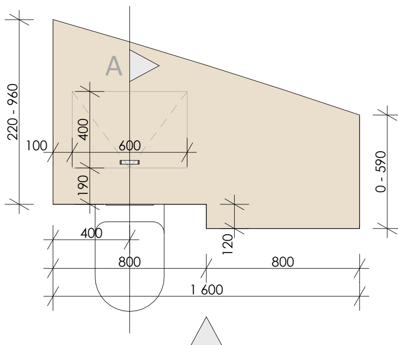
PŮDORYS
