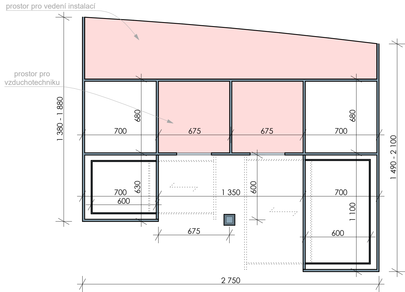
POHLED A
