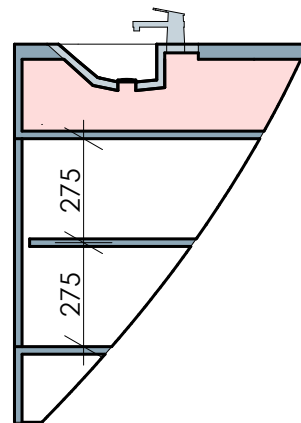
ŘEZ A
