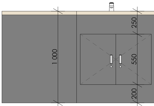
ČELNÍ POHLED
