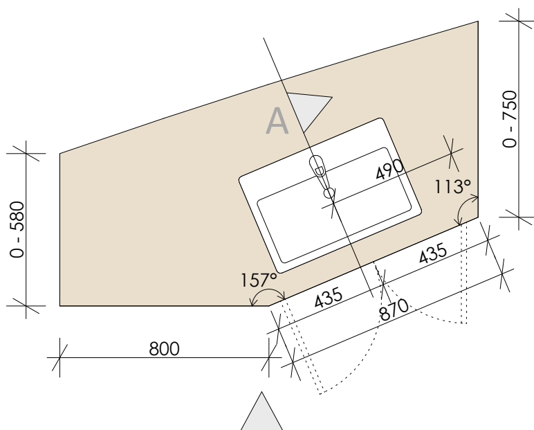
PŮDORYS
