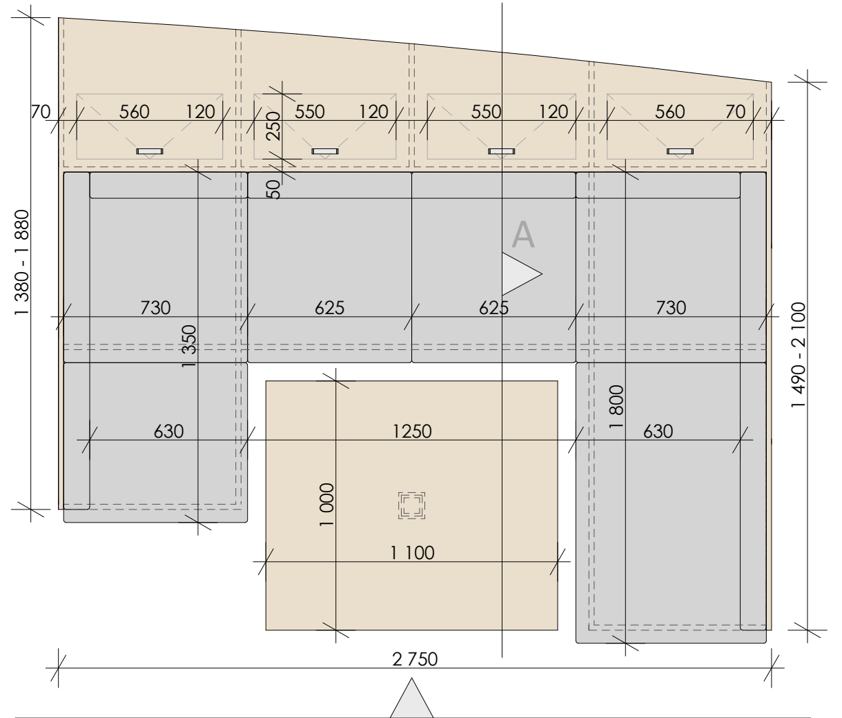
PŮDORYS
