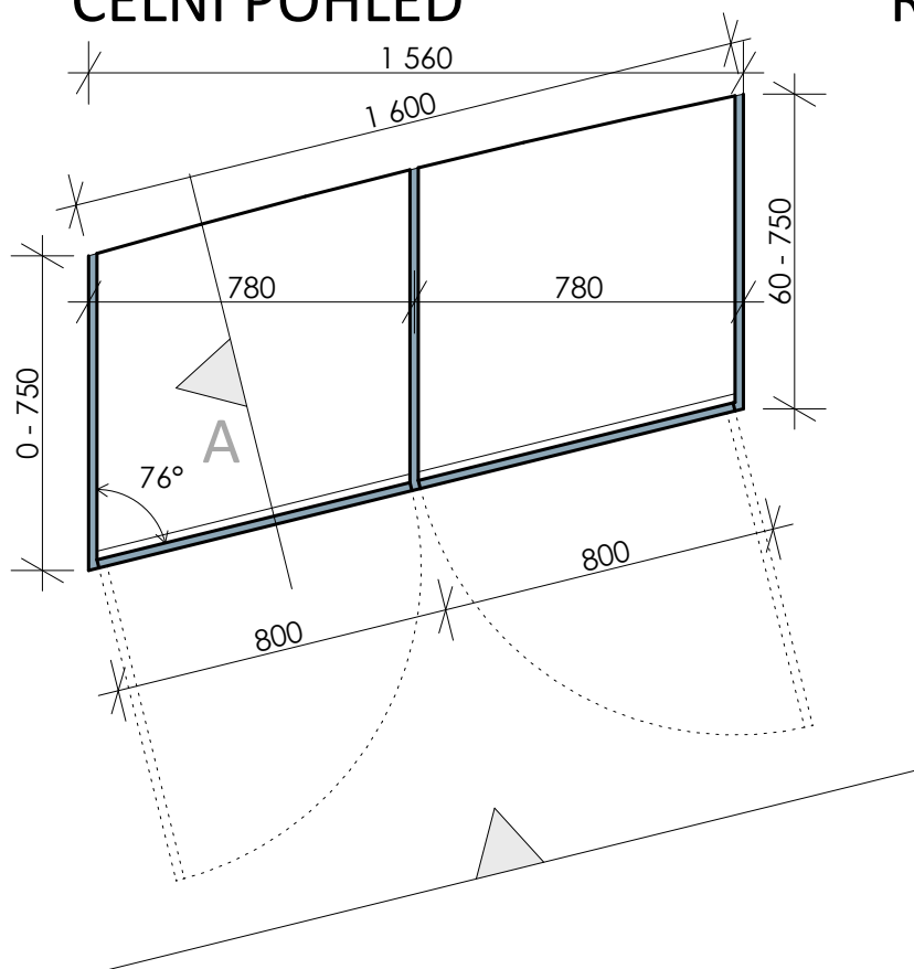
PŮDORYS
