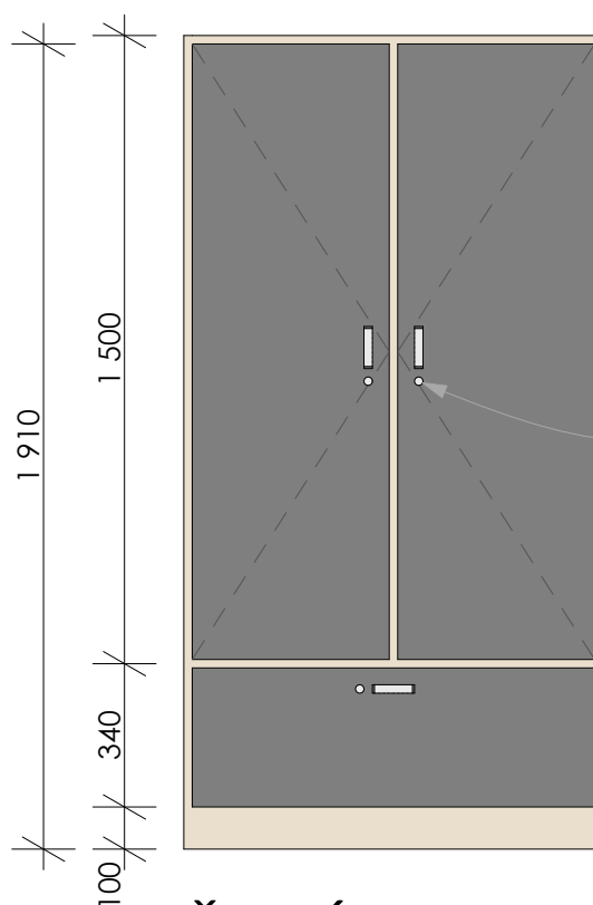
ČELNÍ POHLED
