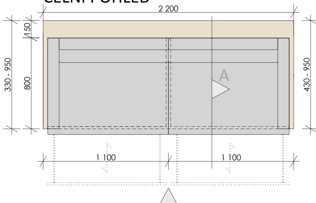
PŮDORYS
