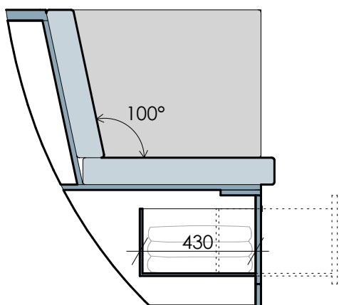
ŘEZ A
