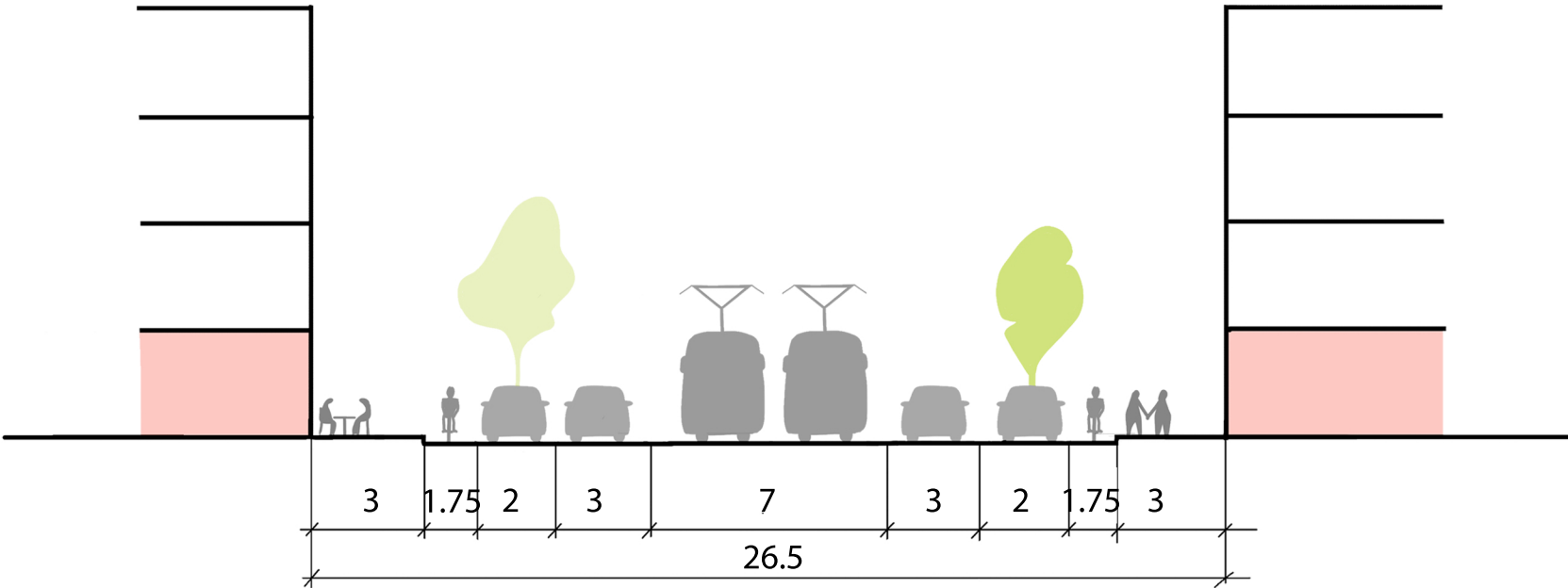
ŘEZ 3-3 M1:50
