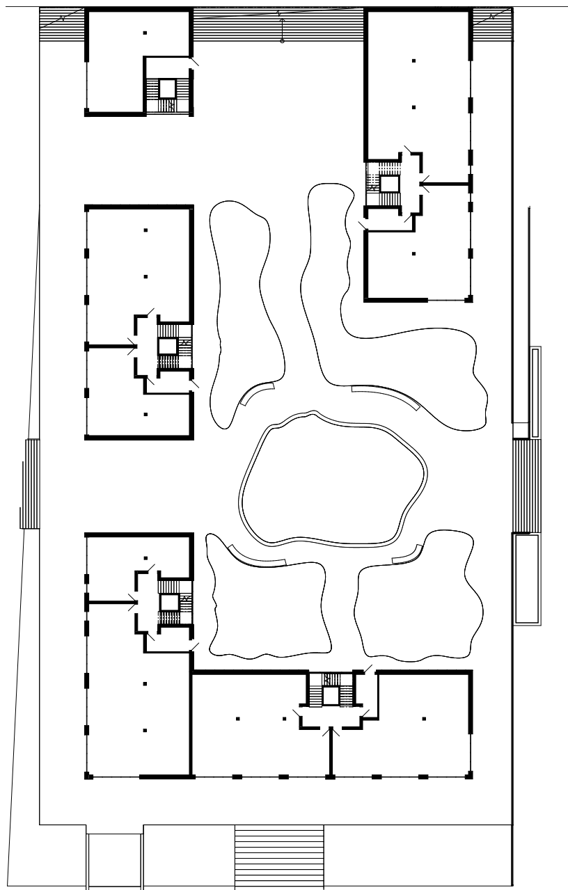
PŮDORYS 1NP
