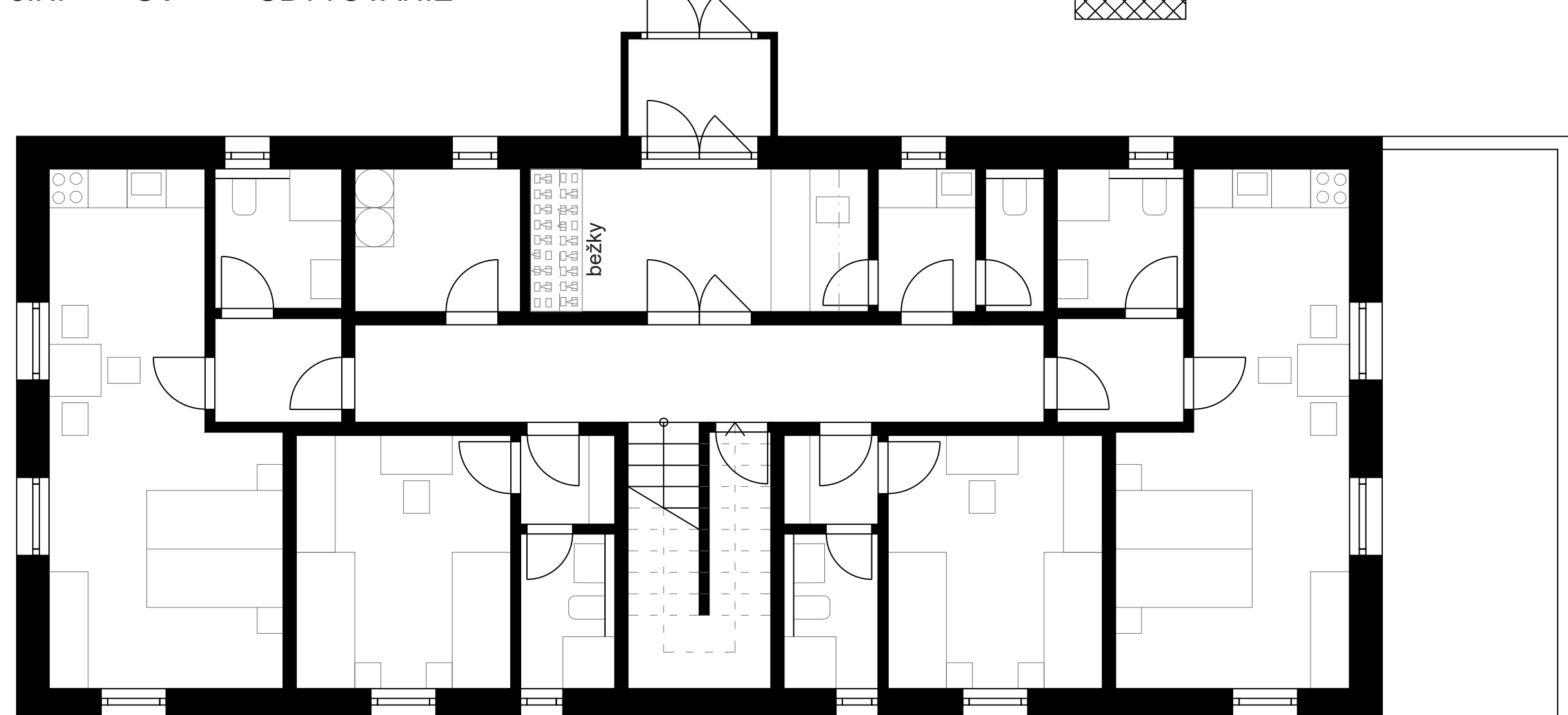
2.NP O1 UBYTOVANIE S RECEPCIU
