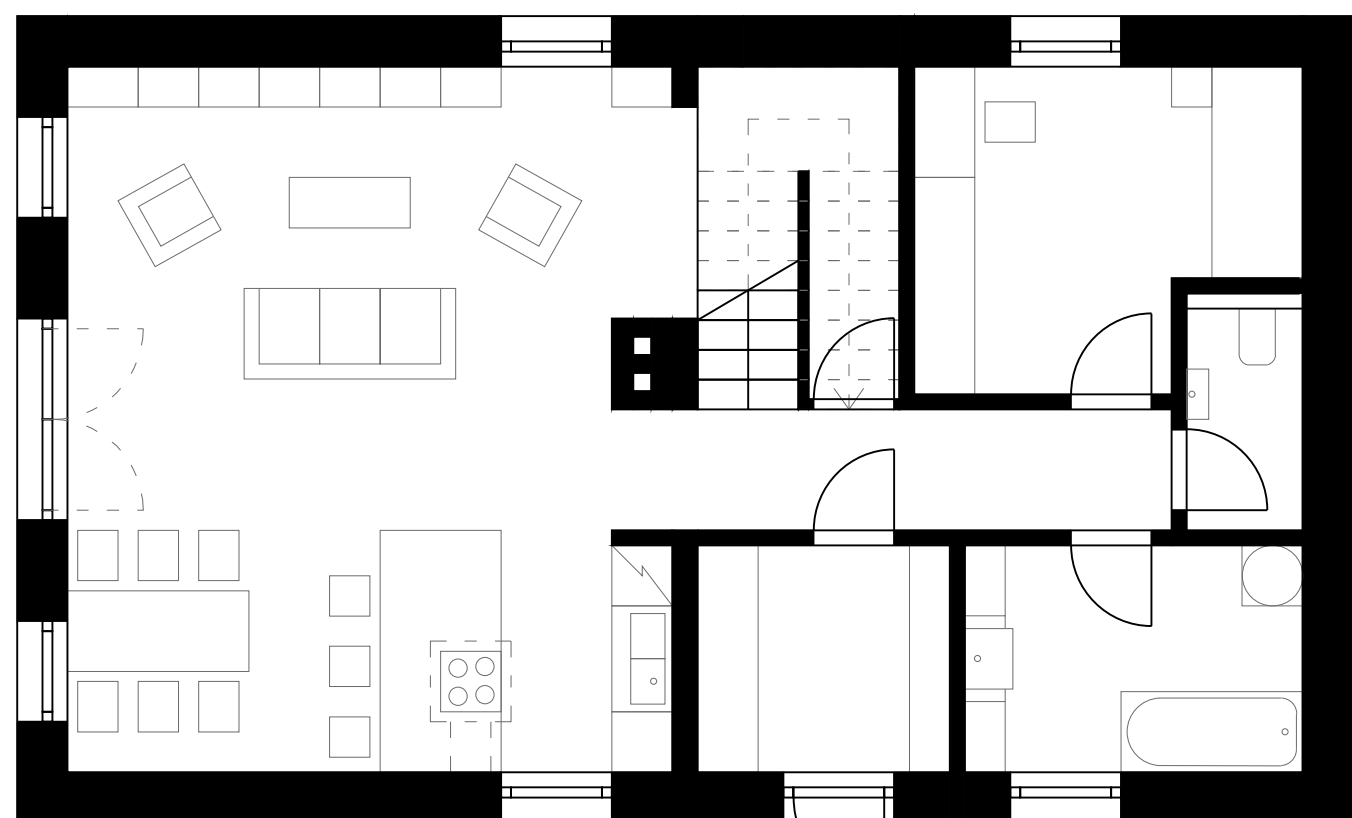
1.NP O3 RODINNÝ DOM SPRÁVCU
