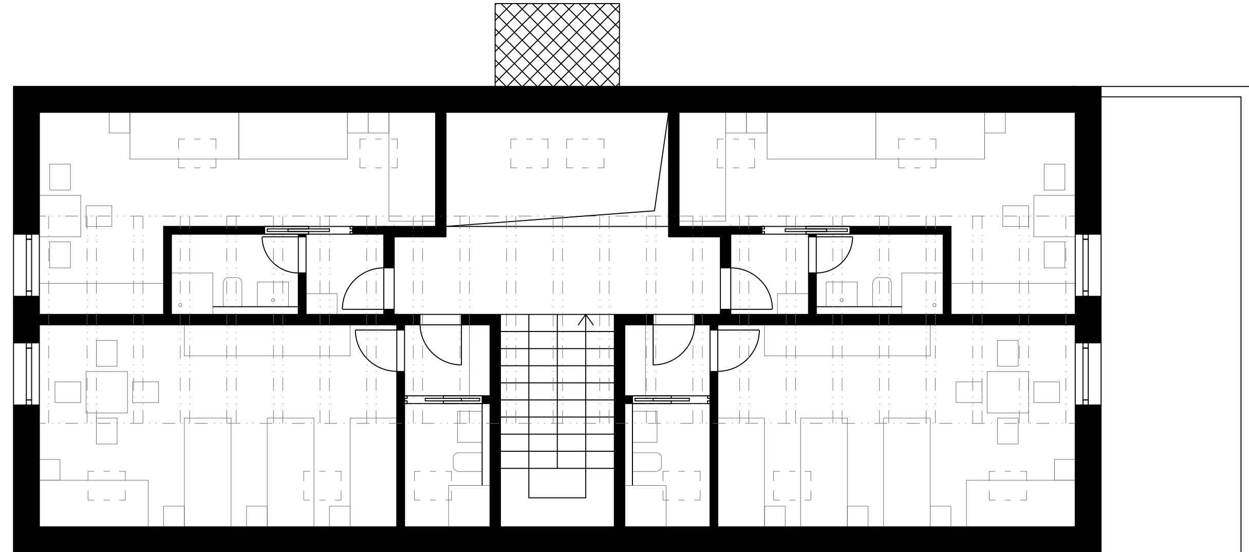
3.NP O1 UBYTOVANIE
