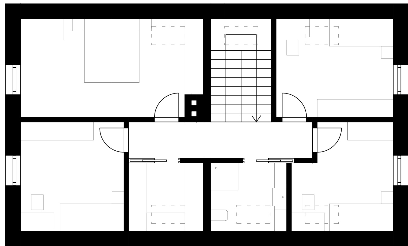
2.NP O3 RODINNÝ DOM SPRÁVCU
