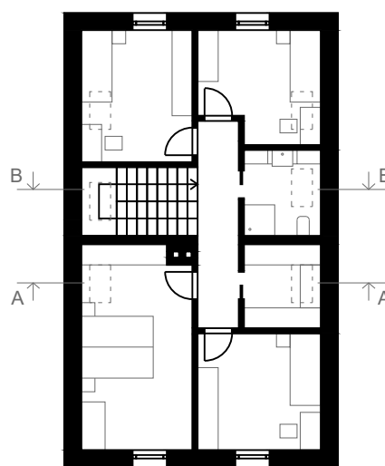
2.NP
