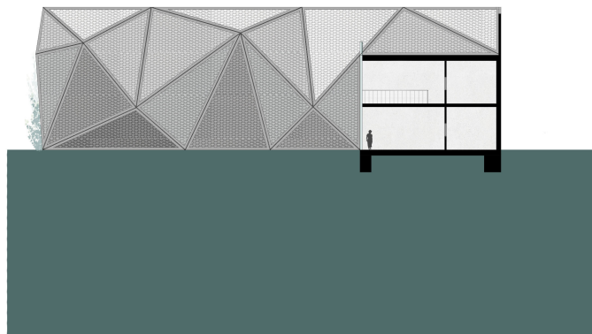
REZ B-B'
