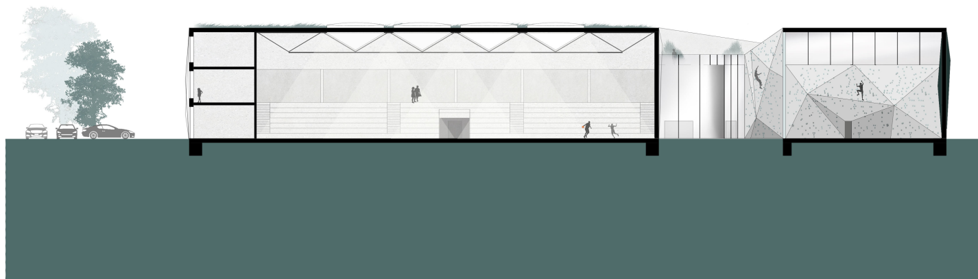
REZ A-A'
