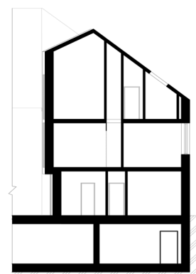
ŘEZ B-B
