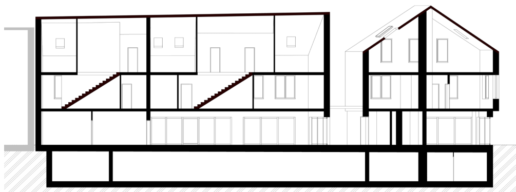
ŘEZ A-A
