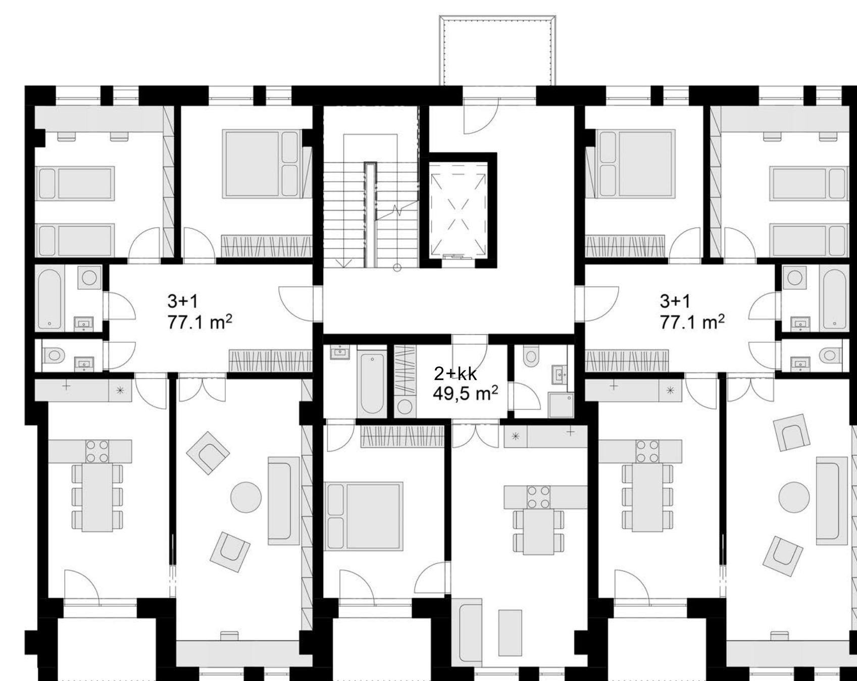
DISPOZICE TYPICKÉ 4 PODLAŽÍ 1:100
