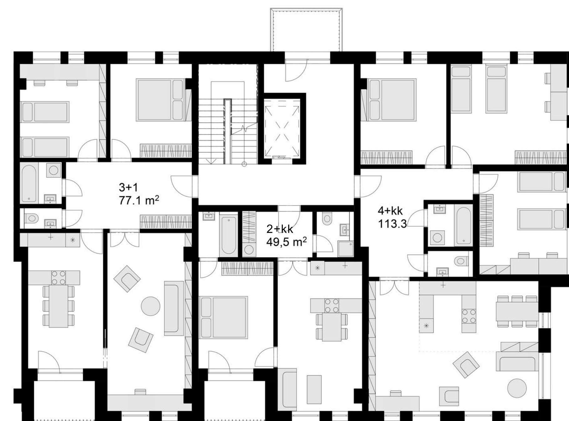
DISPOZICE TYPICKÉ 3 PODLAŽÍ KRAJNÍ SEKCE 1:100
