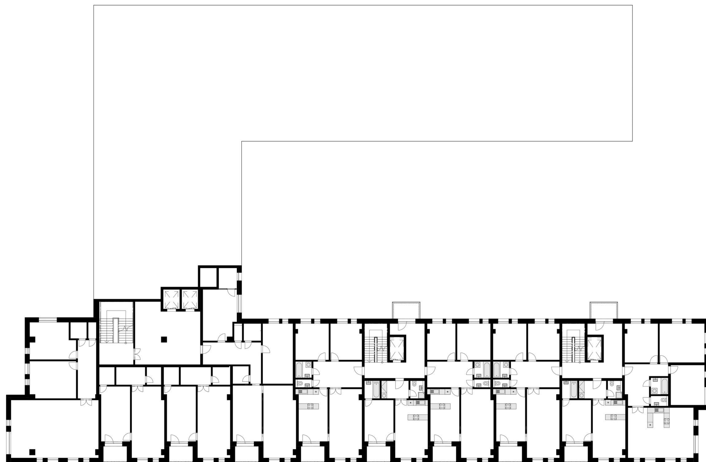
TYPICKÉ 3 PODLAŽÍ 1:200
