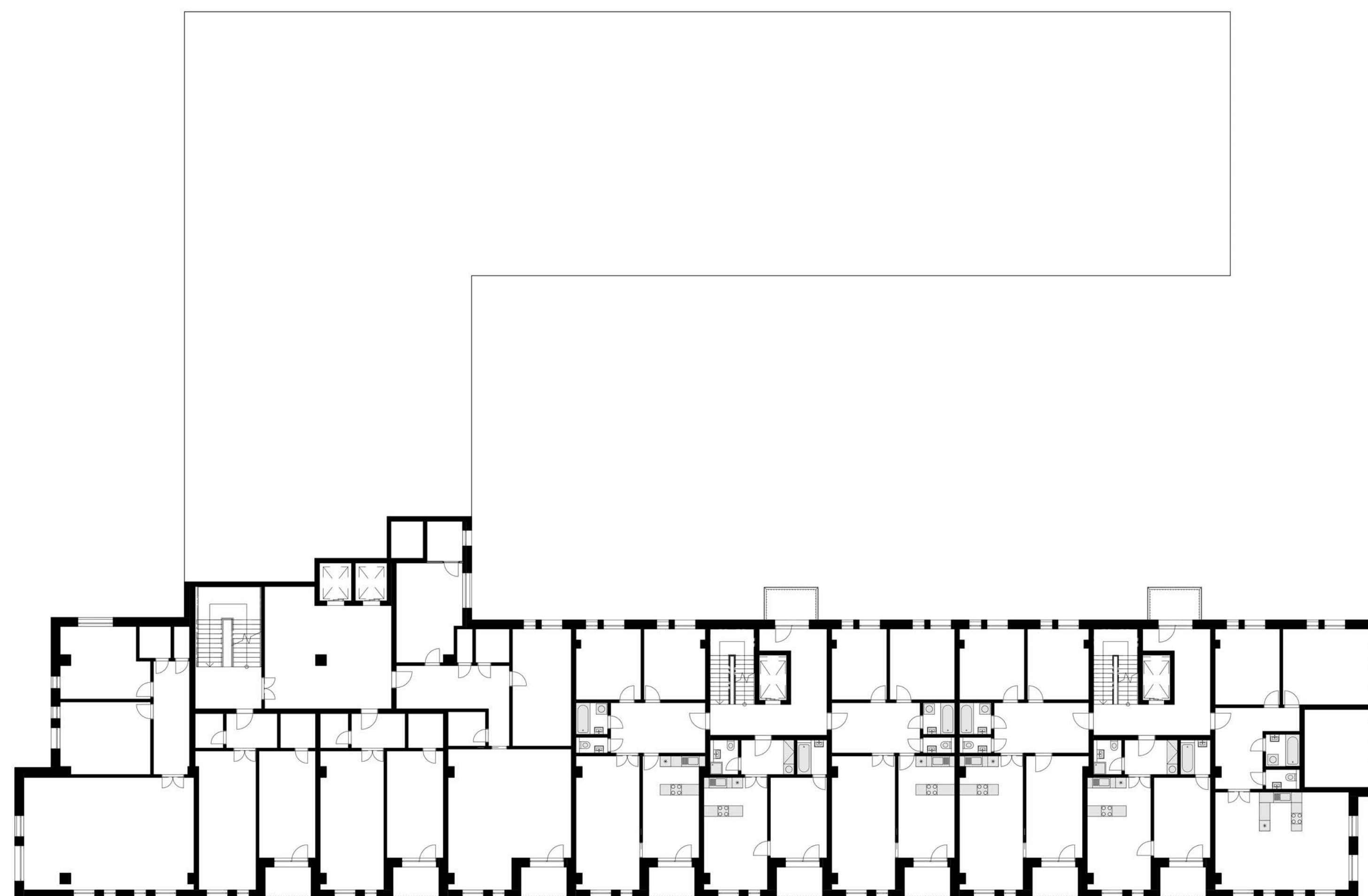
TYPICKÉ 4 PODLAŽÍ 1:200
