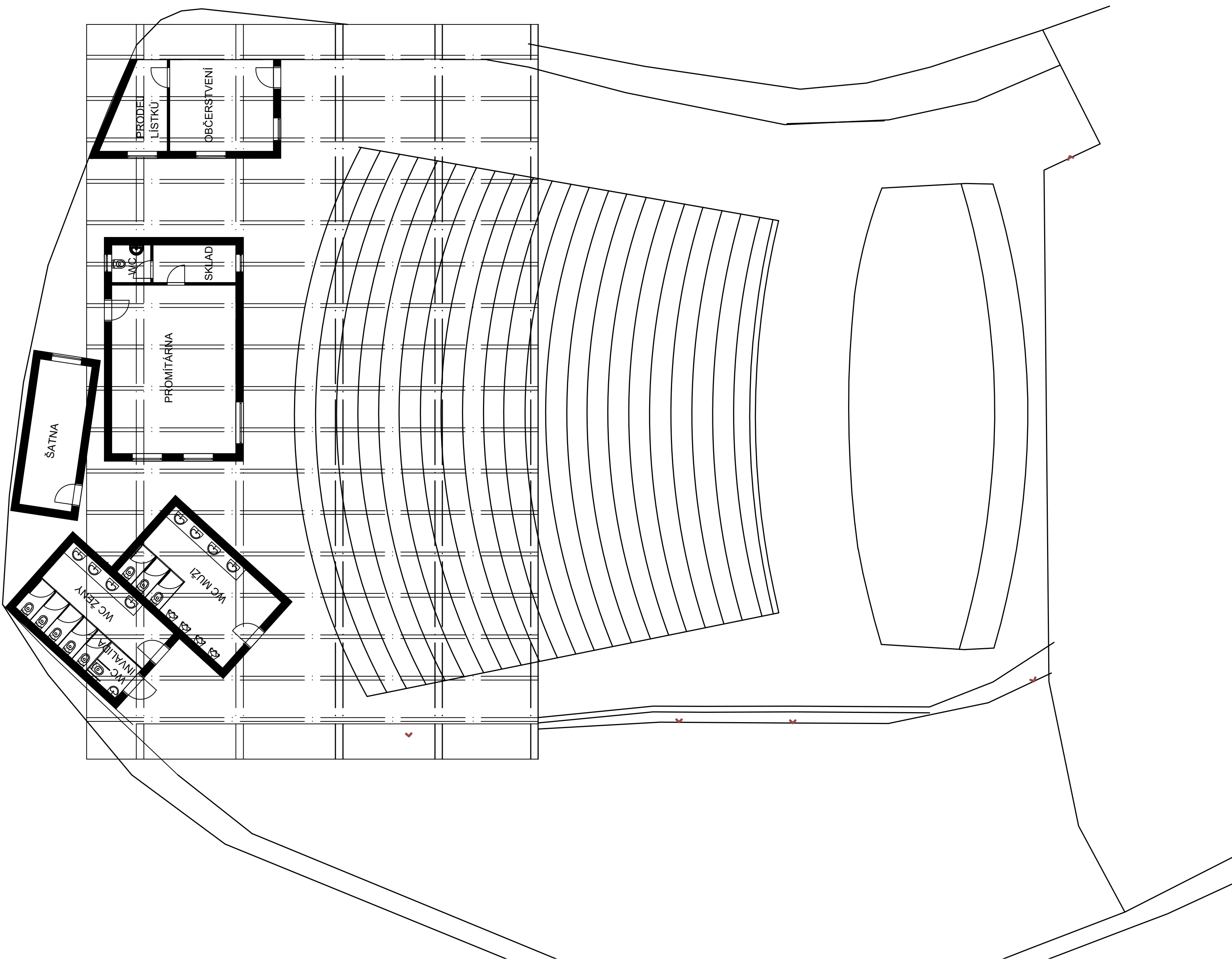
PŮDORVY 1:150
