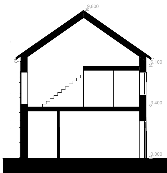
ŘEZ 3_obchod
