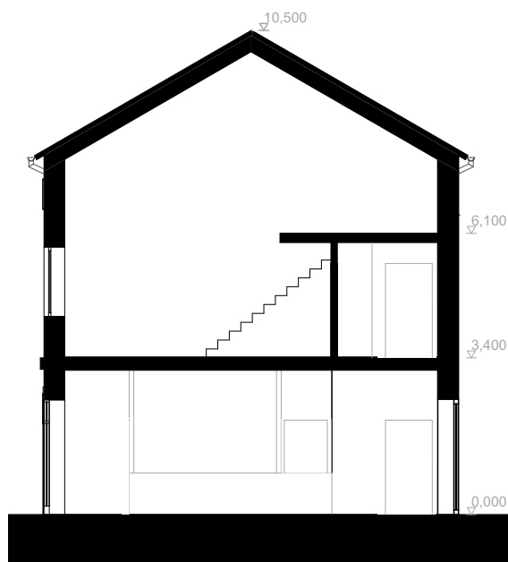
ŘEZ 1_kavárna
