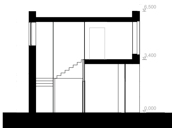
ŘEZ 2_schodiště
