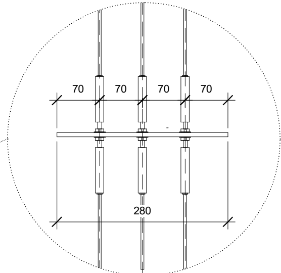
kotvení stupnice
