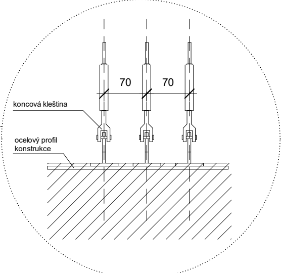
kotvení do betonové podlahy
