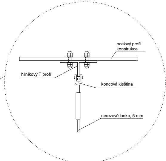
kotvení do konstrukcí nahoře
