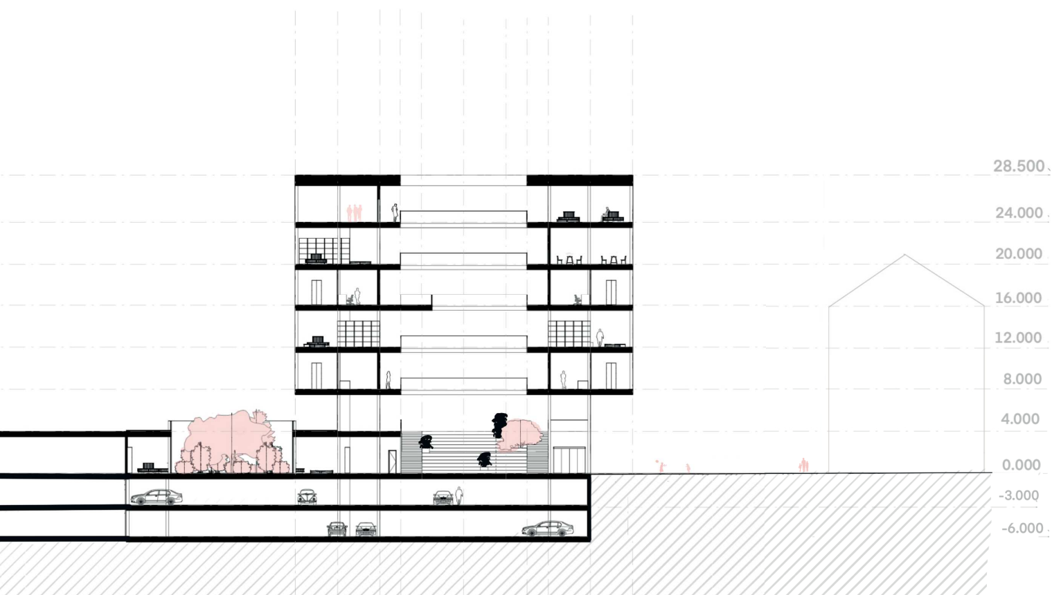
ŘEZ 1:500
