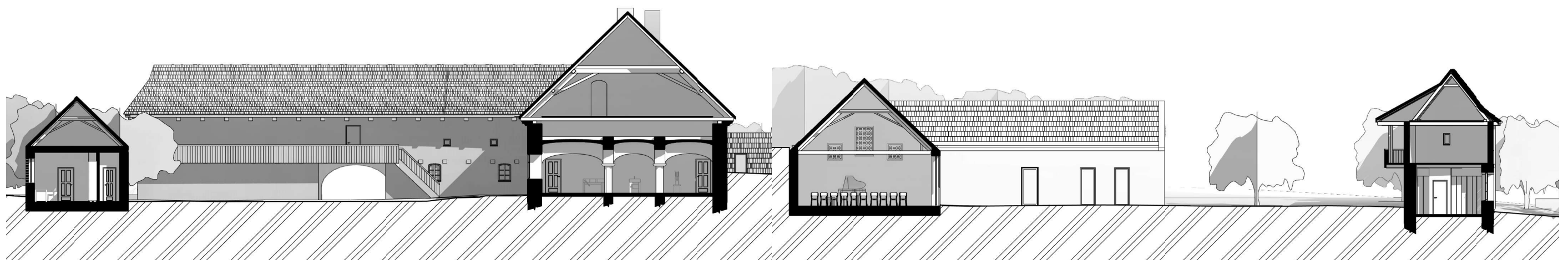
Severní řezopohled
