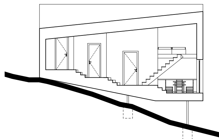
ŘEZ D-D'
