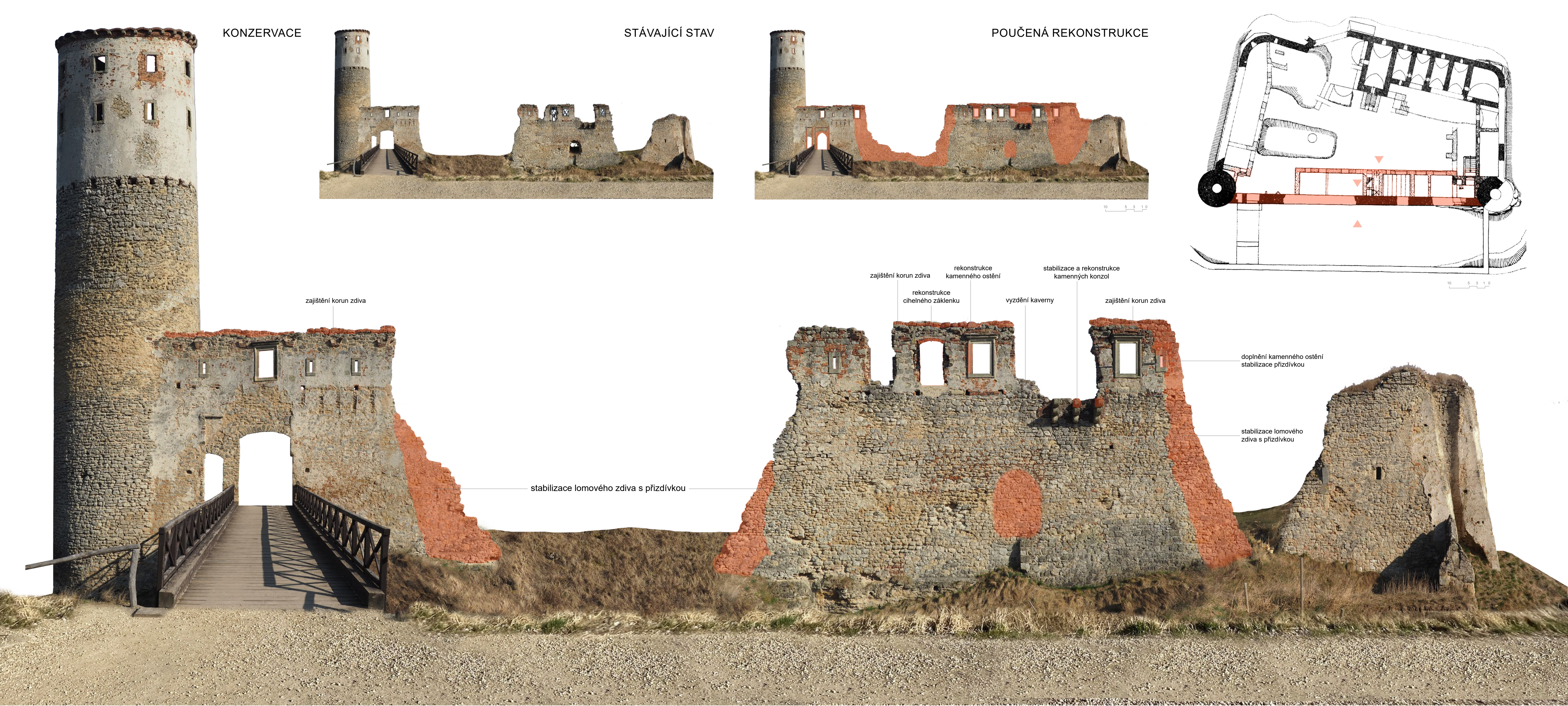
ZÁPADNÍ OBVODOVÁ ZEĎ - POHLED VNĚJŠÍ
