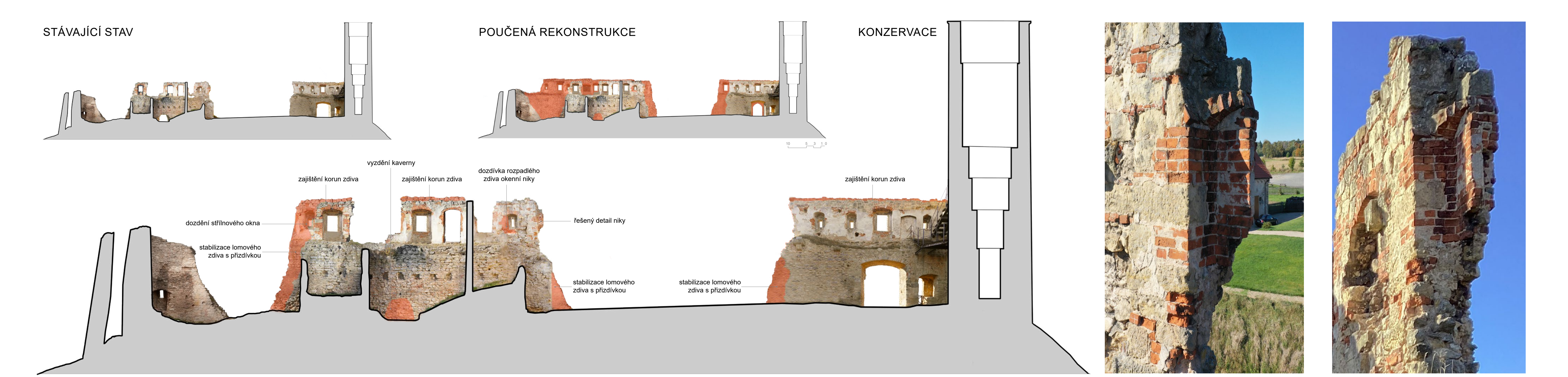
ZÁPADNÍ OBVODOVÁ ZEĎ - POHLED VNITŘNÍ
