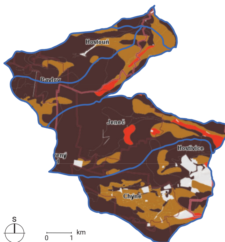
HLOUBKA PŮDY
