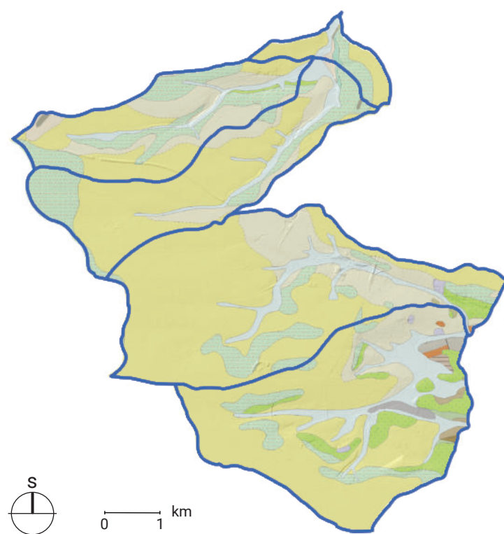
GEOLOGICKÁ MAPA
