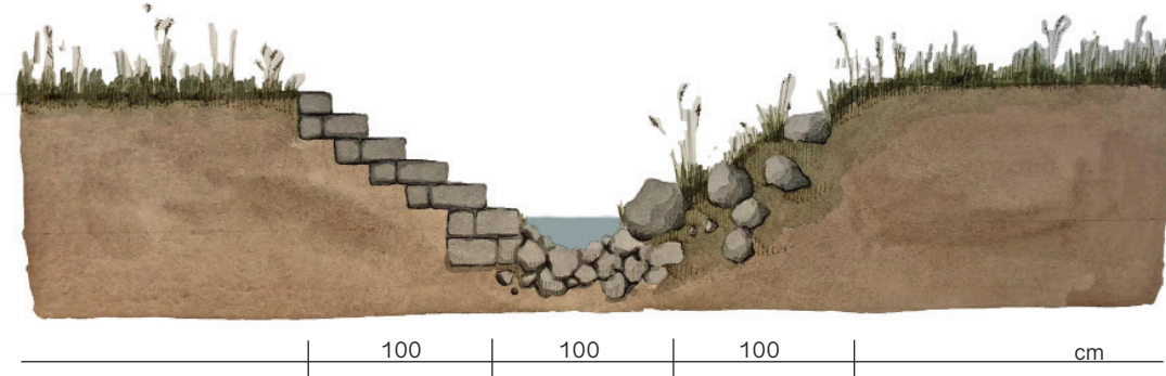
NAVRHOVANÝ STAV
