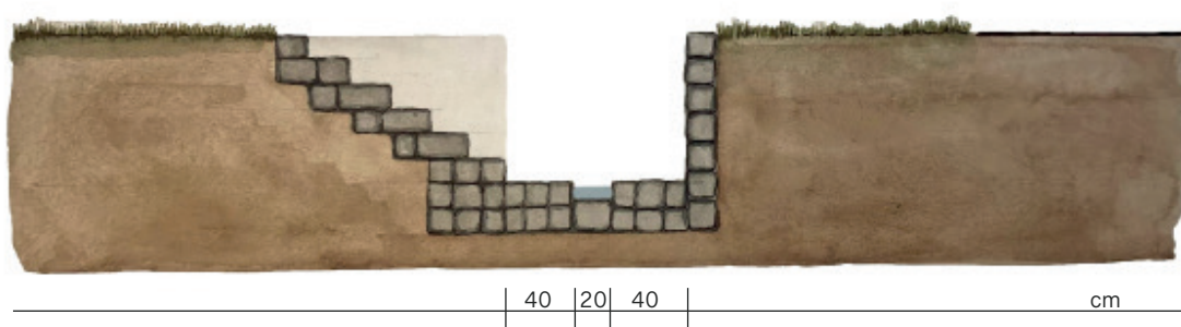
NAVRHOVANÝ STAV
