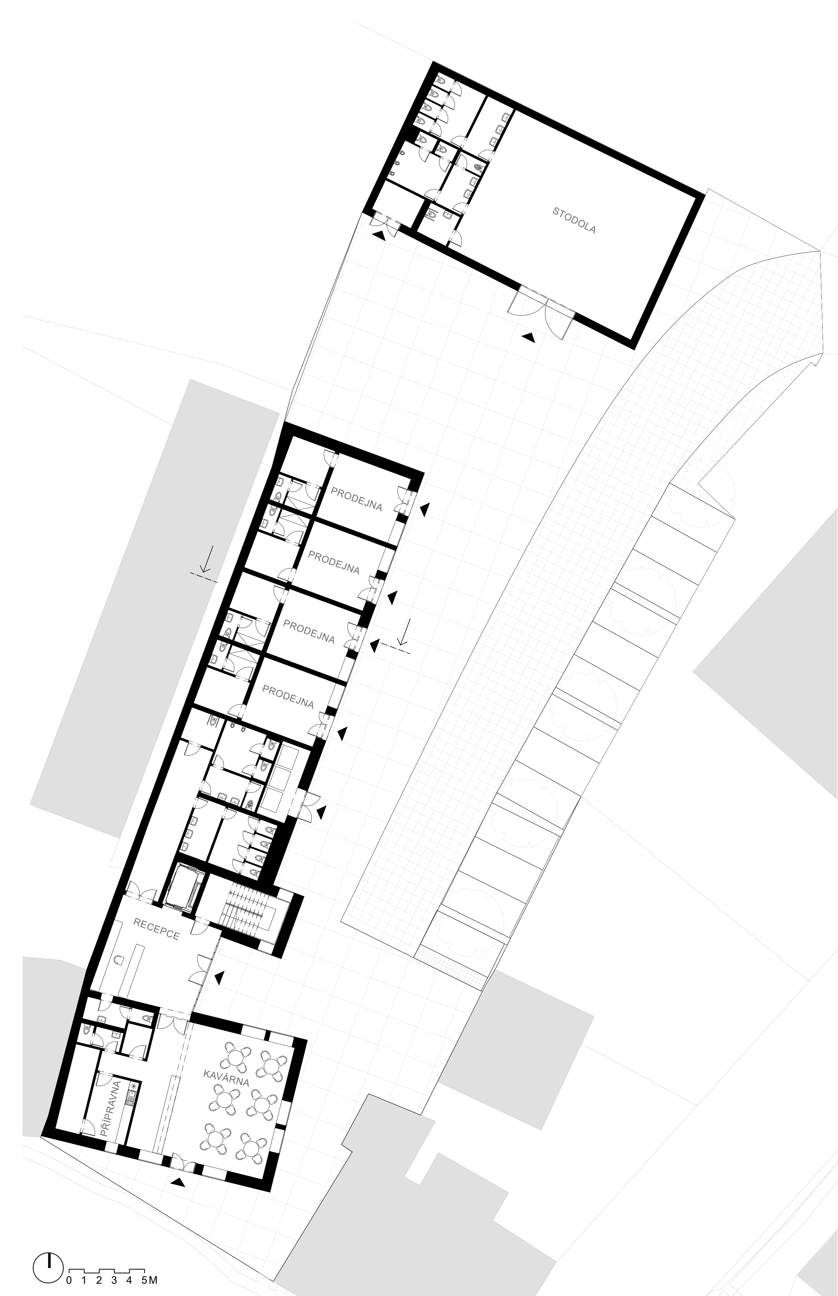
PŮDORYS PRÍZEMÍ M 1:150
