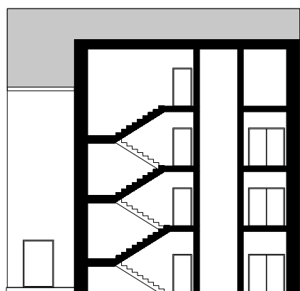
ŘEZ B-B' 1:300
