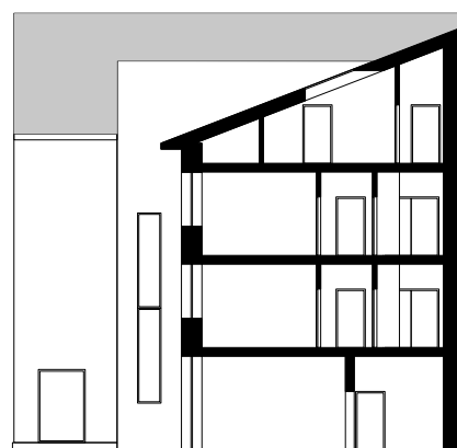
ŘEZ C-C' 1:300
