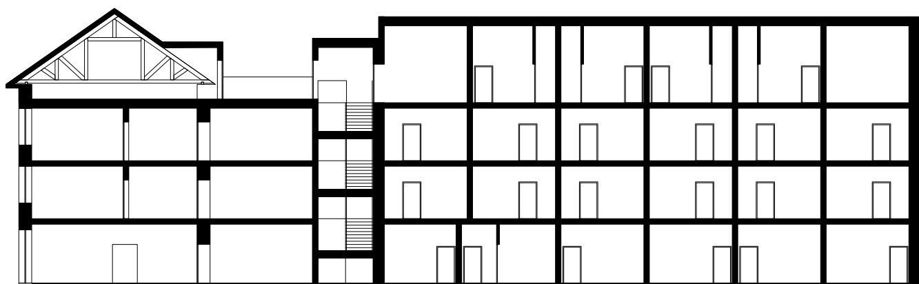
ŘEZ A-A' M 1:300
