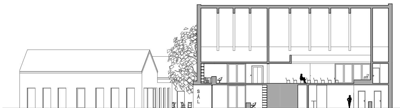
podélný řez
