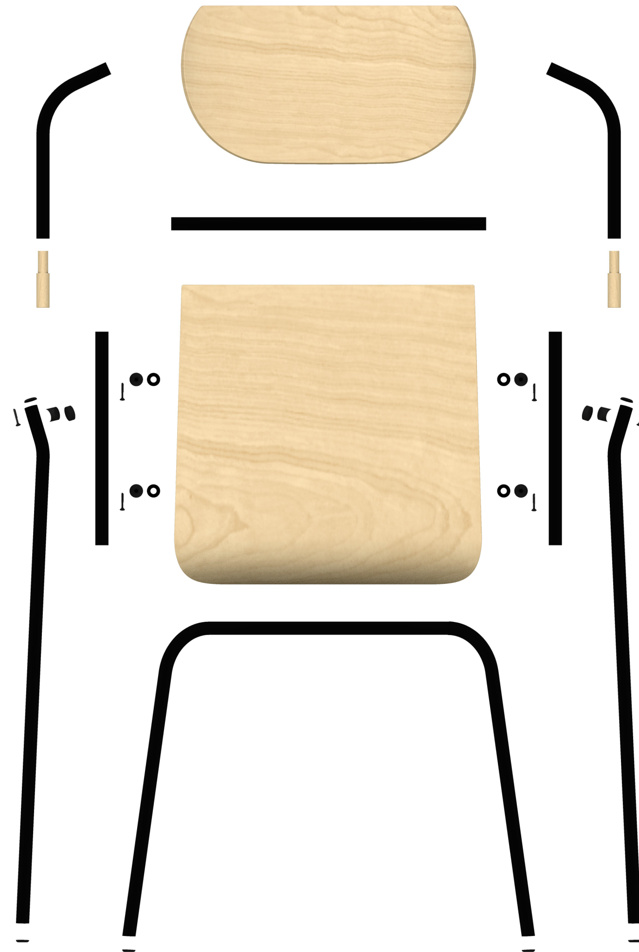
židle POCEM, 1:5 [mm]
