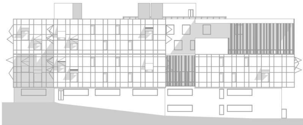
POHLED SV M 1:500
